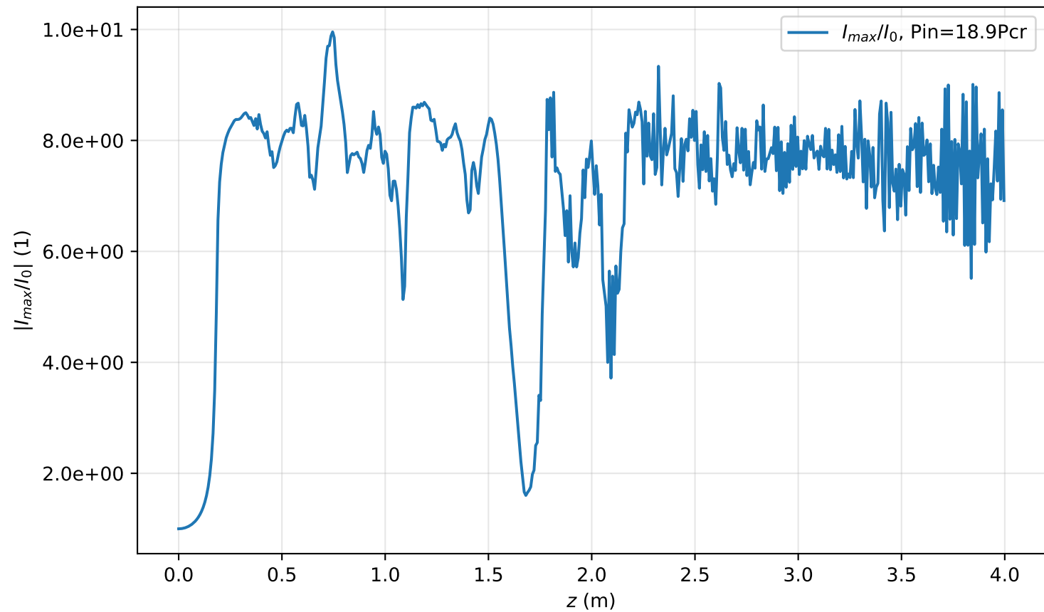
I_{max}(r=0, z)/I_0 , Pin=18.9Pcr
