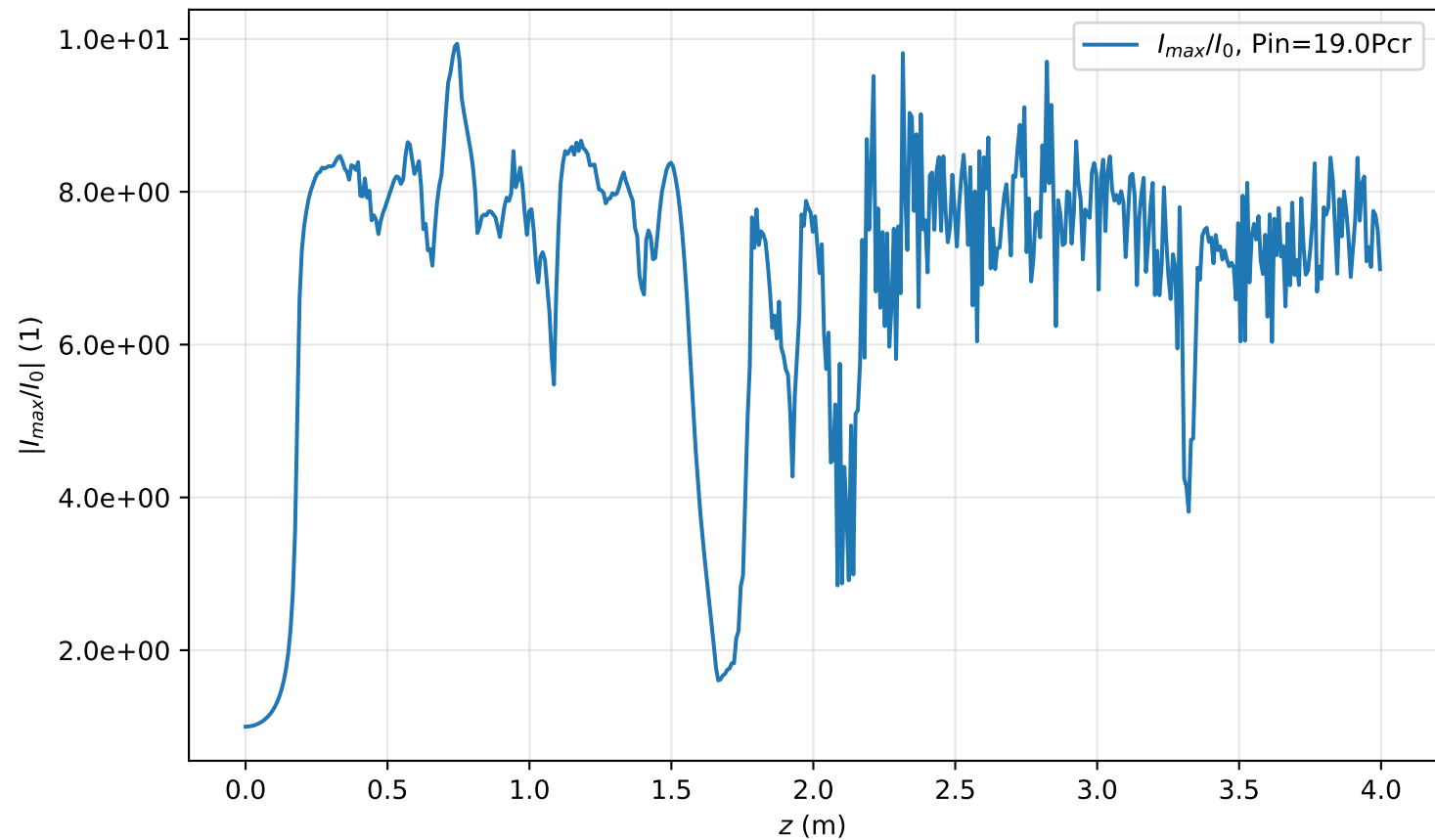
I_{max}(r=0, z)/I_0 , Pin=19.0Pcr
