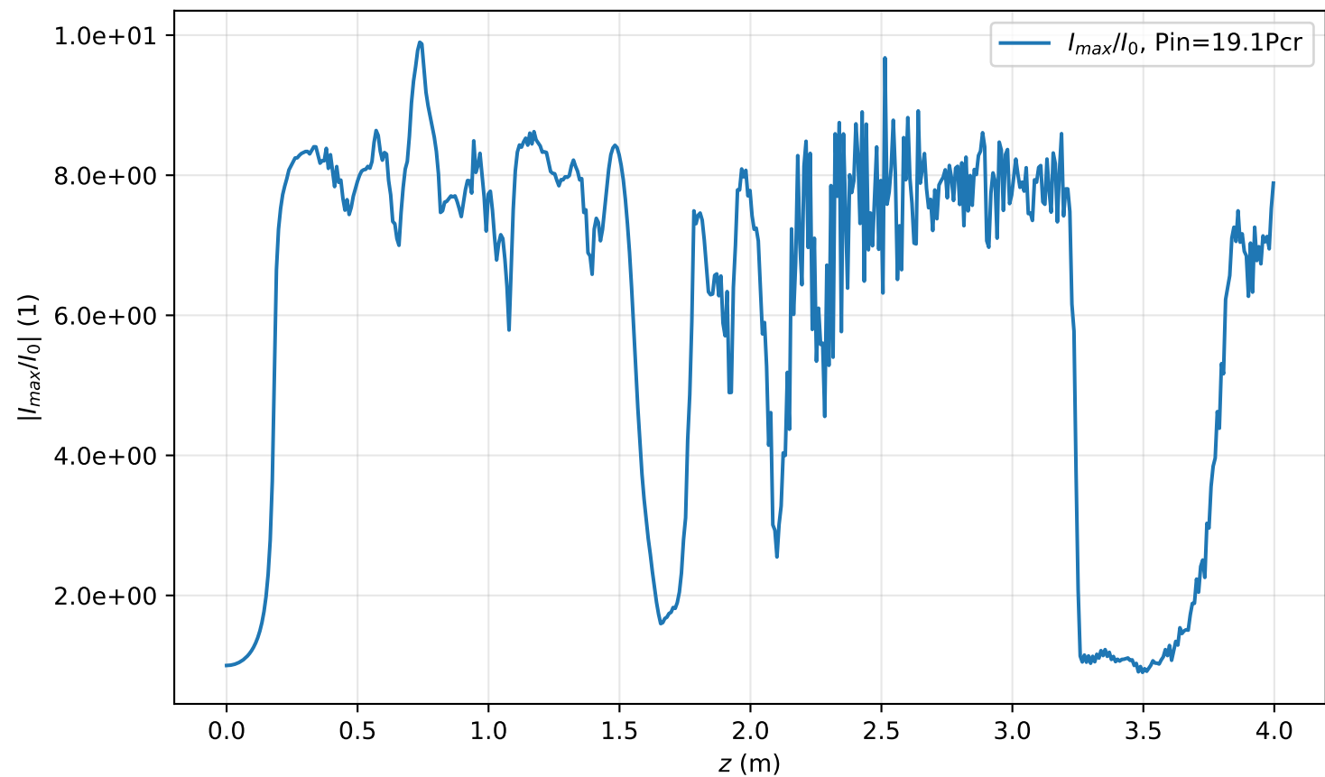
I_{max}(r=0, z)/I_0 , Pin=19.1Pcr
