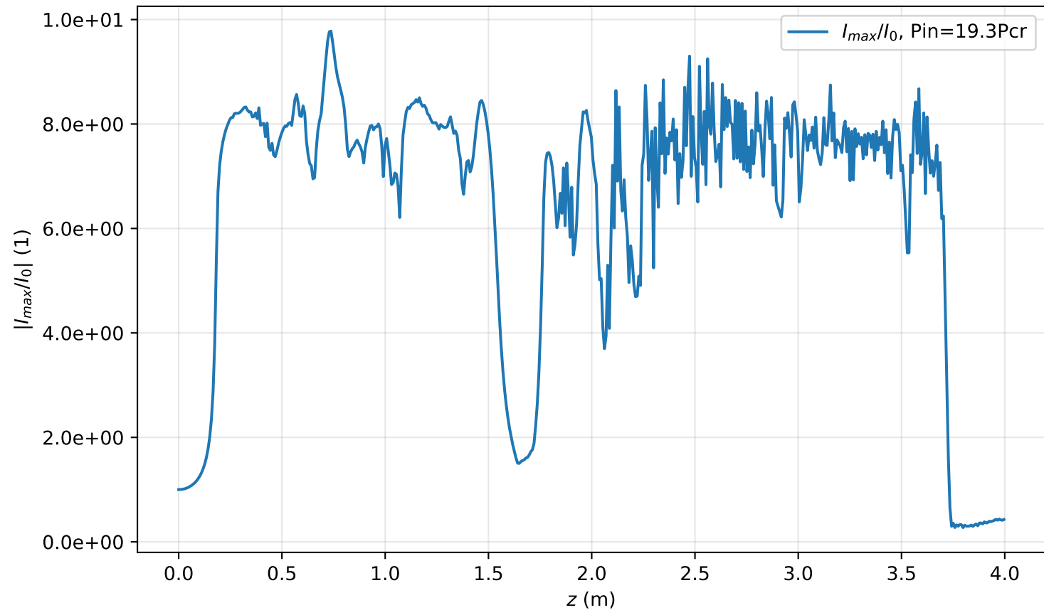
I_{max}(r=0, z)/I_0 , Pin=19.3Pcr
