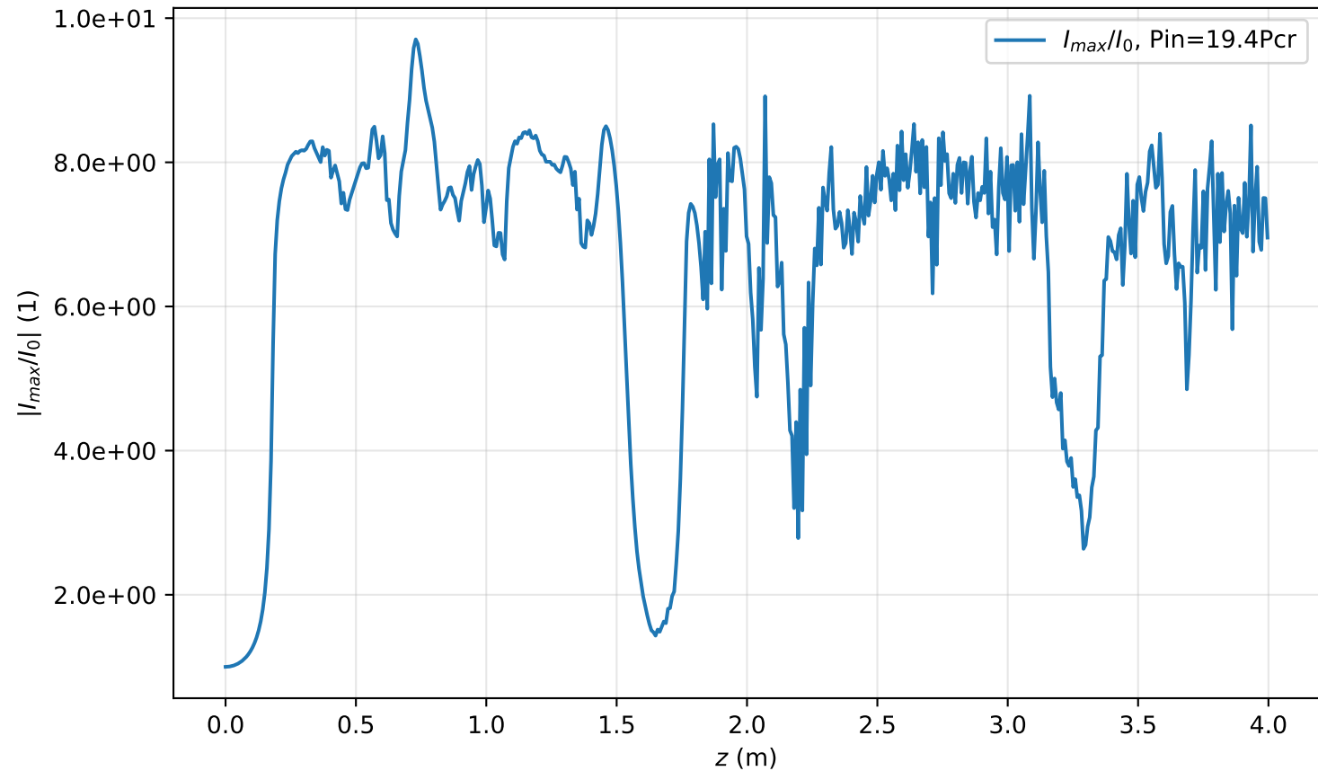
I_{max}(r=0, z)/I_0 , Pin=19.4Pcr
