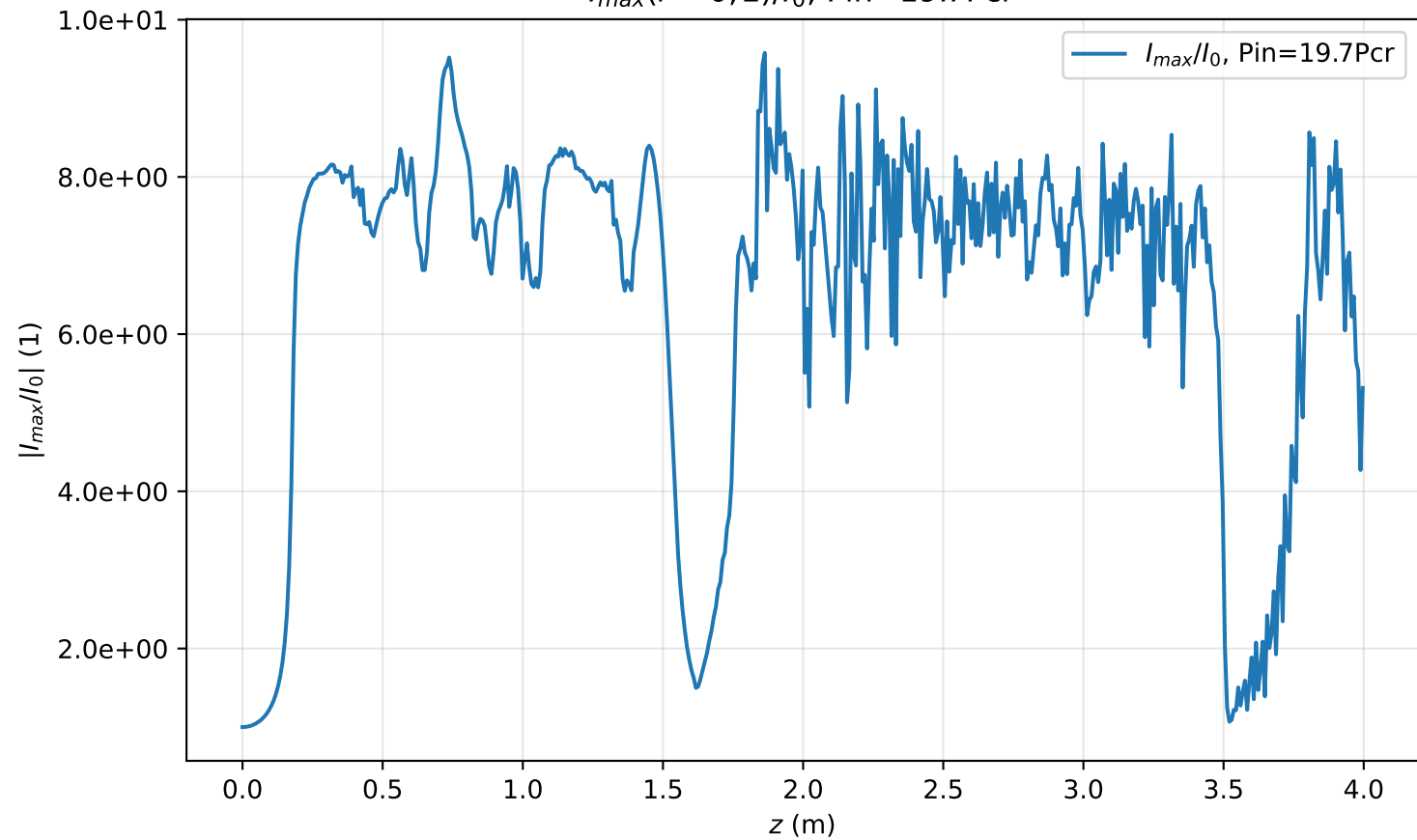
I_{max}(r=0, z)/I_0 , Pin=19.7Pcr
