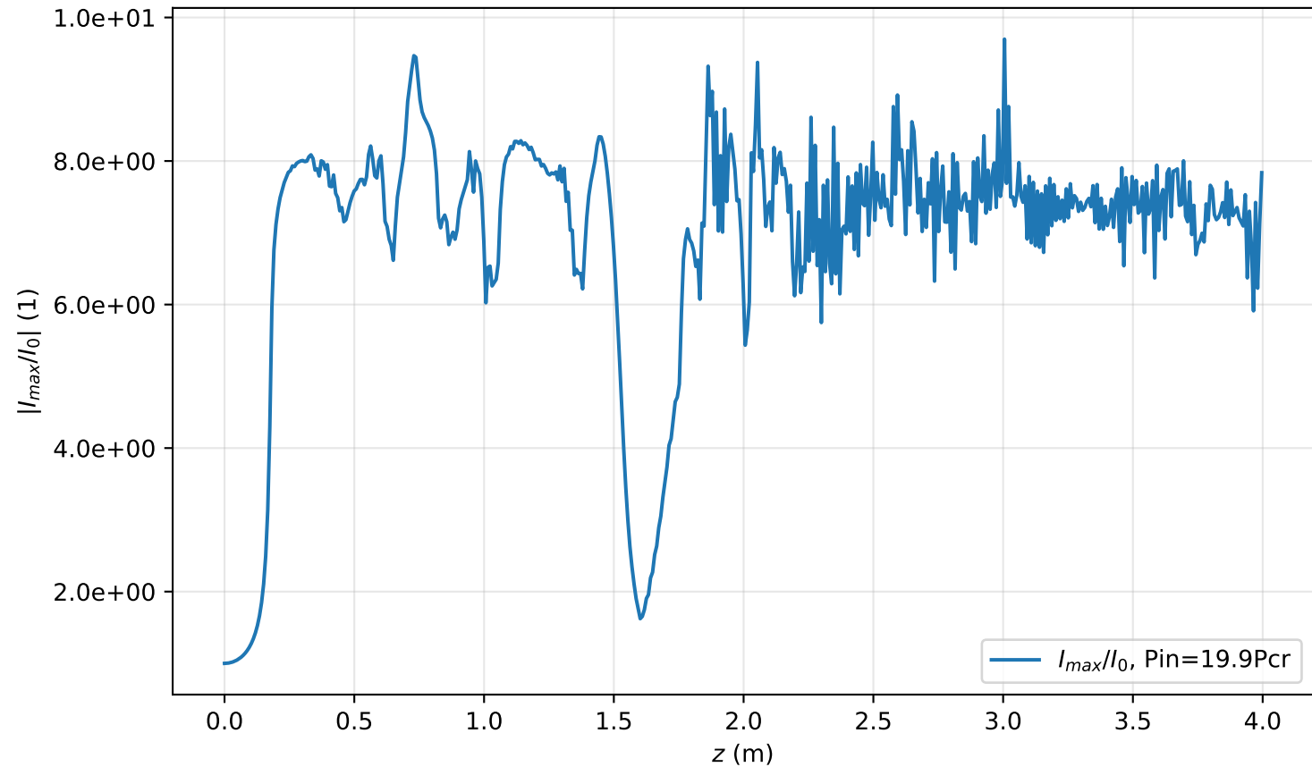
I_{max}(r=0, z)/I_0 , Pin=19.9Pcr
