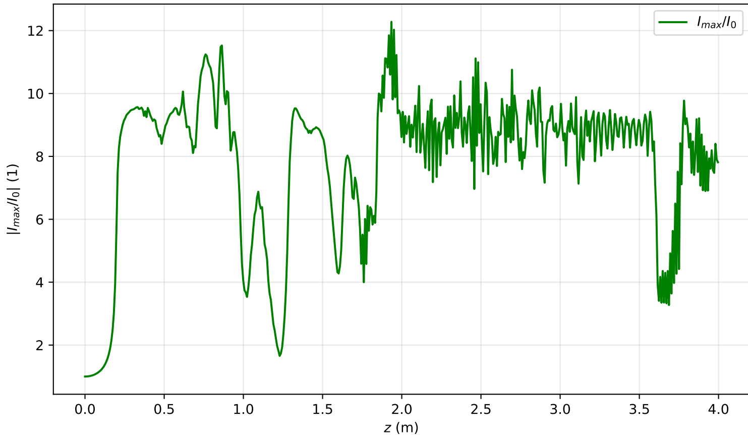
I_{\max}(r=0, z)/I_0 , Pin=16.7Pcr
