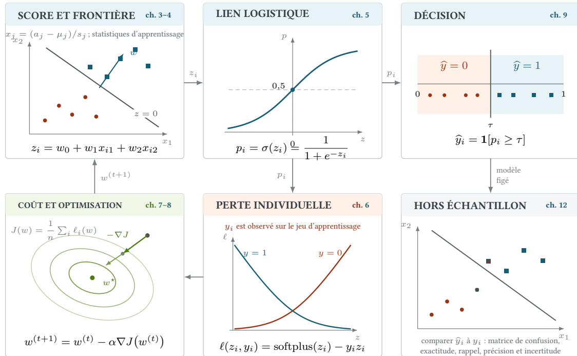
FIGURE 1.1: Vue d'ensemble du modèle. La rangée supérieure transforme une observation en classe prédite pour des coefficients fixés. La rangée inférieure relie l'étiquette observée à la perte, à l'optimisation des coefficients et au contrôle sur un jeu tenu hors de l'ajustement.
