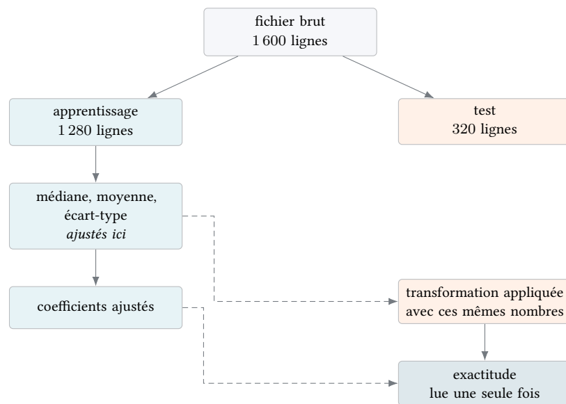
FIGURE 12.2: Les statistiques de préparation sont des paramètres ajustés au même titre que les coefficients. Les flèches en pointillé transportent des nombres figés, jamais un nouvel ajustement.
