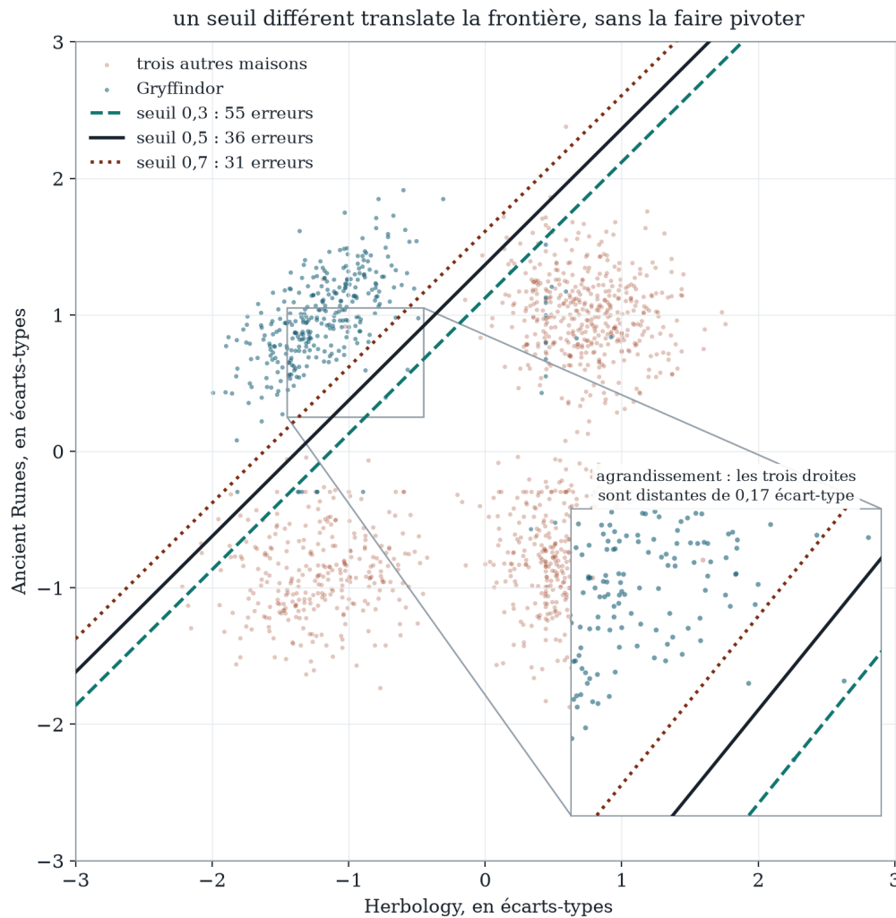
FIGURE 12.6: Nuage standardisé et droites des seuils 0,3, 0,5 et 0,7 : même direction, biais décalés. L'agrandissement porte les observations qui changent de réponse d'une droite à l'autre.
