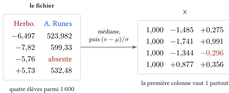
FIGURE 10.2: La médiane d' Ancient Runes , 463,92, remplace la note absente de la troisième ligne et donne -0,296 après standardisation. Les six nombres employés proviennent de fit_stats .
