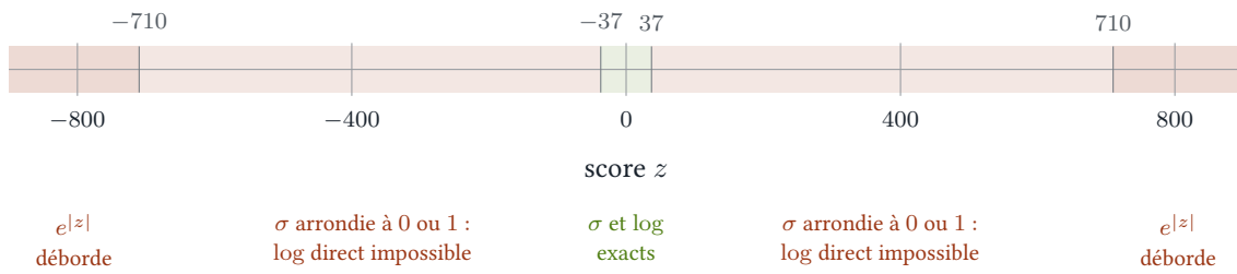
FIGURE J.1: Trois régimes du calcul en double précision. L'écriture directe tient dans la zone centrale ; les formes protégées restent finies sur tout l'axe.
