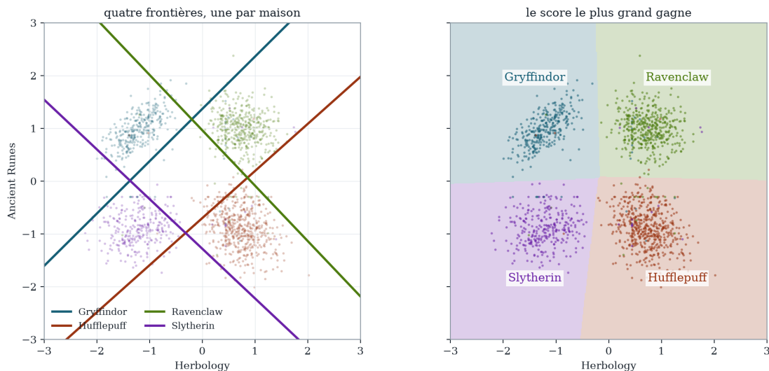
FIGURE 9.2: À gauche, les quatre frontières binaires. À droite, le découpage du plan par la règle du score maximal; les limites entre régions ont leur propre direction.
