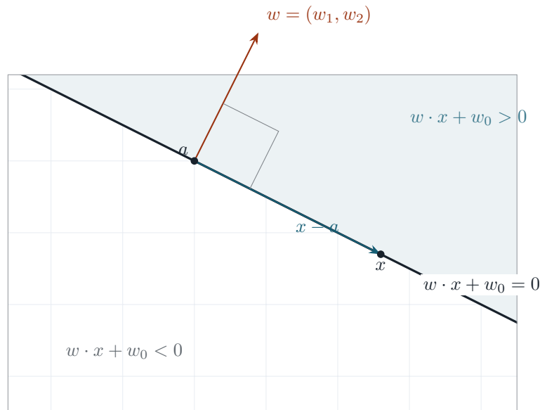
FIGURE 4.3: La droite est l'ensemble des points x tels que x - a soit perpendiculaire à w . Le vecteur w pointe vers le demi-plan où l'expression w \cdot x + w_0 est positive.
