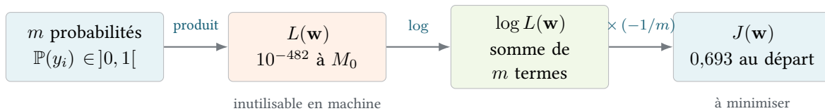
FIGURE E.1: Le produit des probabilités individuelles mesure la plausibilité du jeu de coefficients. Le logarithme le convertit en somme à optimum inchangé ; le facteur -1/m change la maximisation en minimisation et rend la valeur indépendante de l'effectif.
