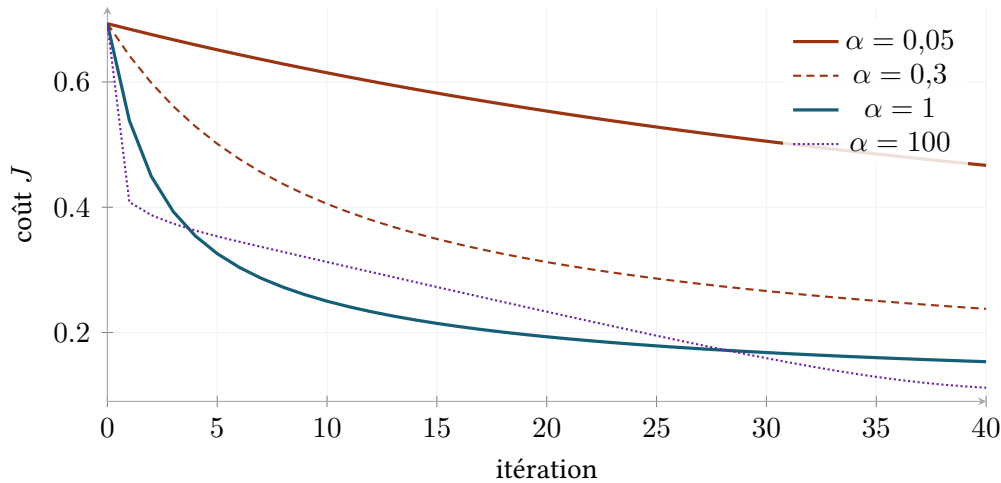
FIGURE I.4: Quarante itérations à partir de M_0 , quatre réglages du pas. À \alpha = 100 , la trajectoire est heurtée : le déplacement dépasse le minimum le long de plusieurs directions.
