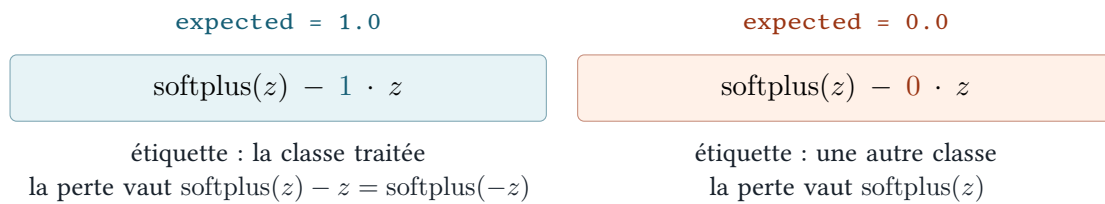
FIGURE 10.3: Les deux cas de la forme stable. L'étiquette intervient dans un terme linéaire au lieu d'un logarithme, ce qui rend l'expression finie pour tout score.
