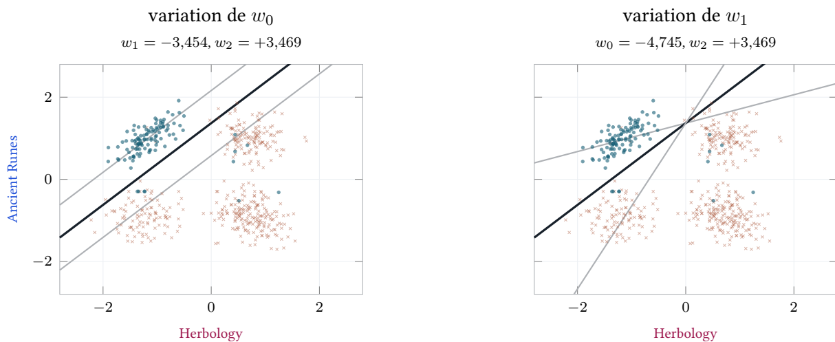
FIGURE 8.1: Variation isolée du biais, à gauche : translation. Variation isolée de w_1 , à droite : rotation et modification de la pente de la sigmoïde.
