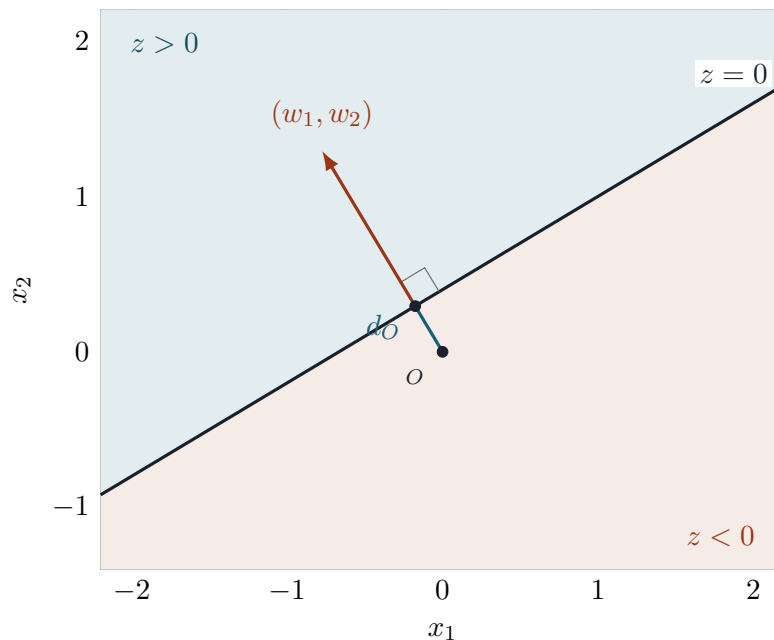
FIGURE K.2: Frontière -0,4 - 0,6x_1 + x_2 = 0 et son vecteur normal (-0,6 ; 1) , tracé à l'échelle depuis le pied de la perpendiculaire issue de l'origine. Le segment d_O mesure -w_0/\|w\| = 0,343 .
