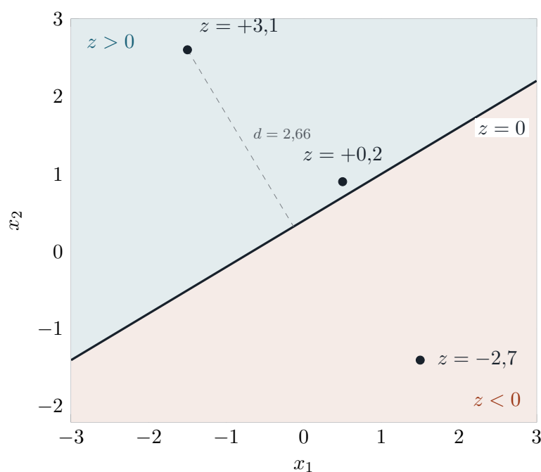
FIGURE 4.4: Frontière pour w = (-0,4; -0,6; 1) . Les distances orthogonales des points de scores +3,1 et +0,2 valent respectivement 2,66 et 0,17 .
