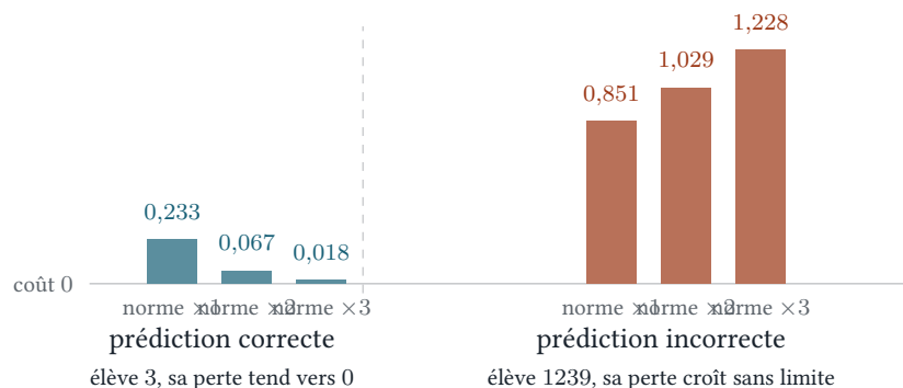
FIGURE H.1: Perte de deux prédictions quand la norme est multipliée par 1, 2 puis 3, à frontière fixe. La perte tend vers zéro pour l'observation correctement classée et croît sans borne pour l'autre.
