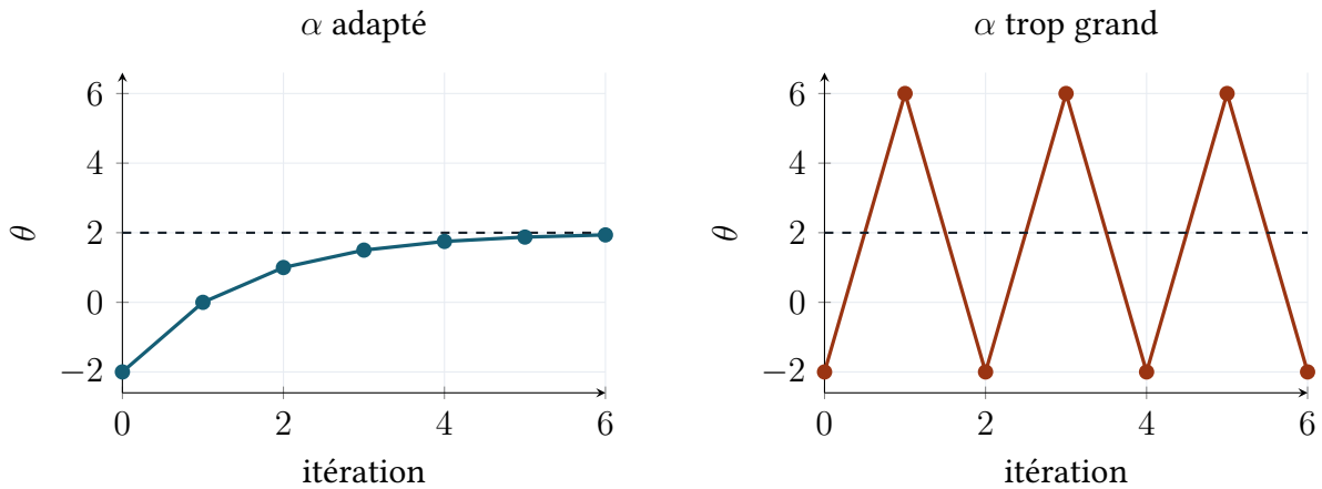
FIGURE I.5: Quadratique d'une variable, courbure c , minimum en 2. À gauche \alpha < 2/c : convergence. À droite \alpha = 2/c : oscillation entre deux valeurs; tout \alpha > 2/c diverge.
