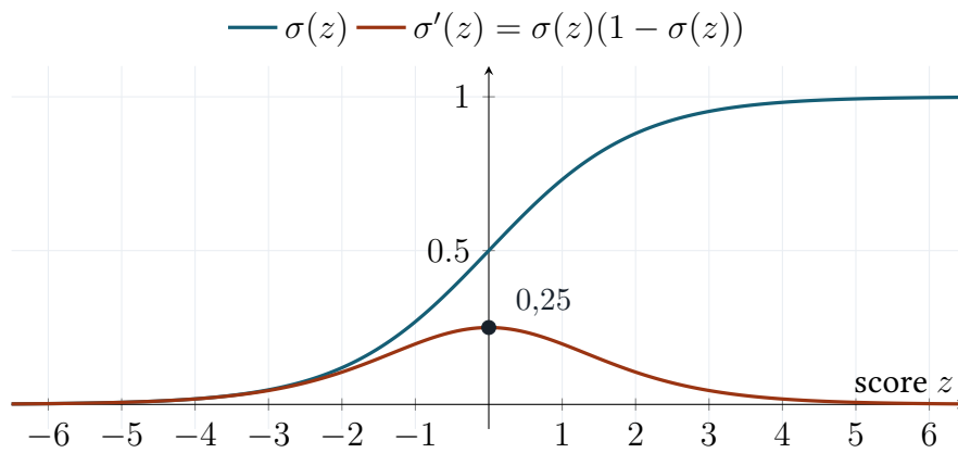
FIGURE D.1: La dérivée atteint son maximum, 0,25, en z = 0 , et tend vers zéro dès que la probabilité approche 0 ou 1.
