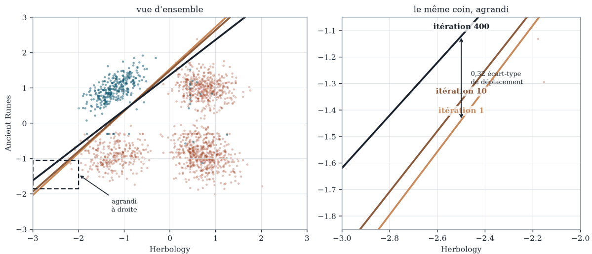
FIGURE 7.2: Frontière aux itérations 1, 10 et 400 ; le rectangle agrandi sépare les trois droites. Elles pivotent autour d'un point central du nuage, pour un déplacement total d'un tiers d'écart-type.
