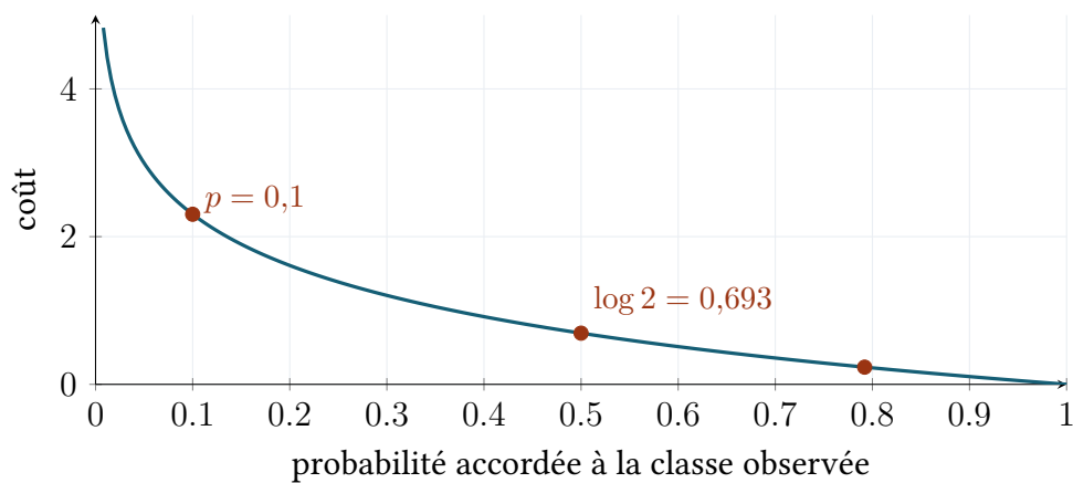
FIGURE 6.1: Perte associée à une prédiction. Elle vaut \log 2 en 0,5, tend vers zéro à droite et croît sans borne à gauche.
