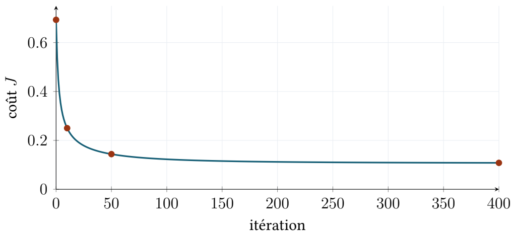
FIGURE 7.1: Perte moyenne aux itérations 0, 10, 50 et 400. Les dix premiers tours couvrent 75,7 % de la baisse totale ; les 350 derniers, 6 %.
