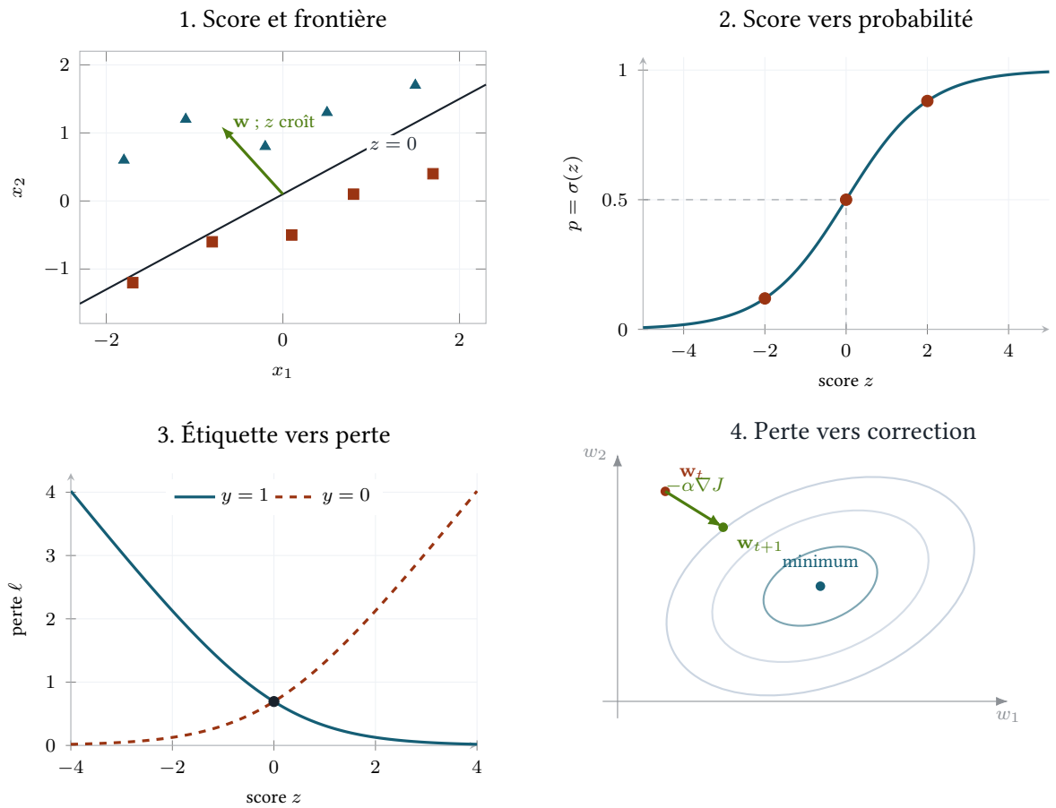
FIGURE 2.1: Vue globale. Le score affine fixe la frontière ; la sigmoïde lui associe une probabilité ; l'étiquette sélectionne une perte ; la moyenne des pertes définit la surface dont le gradient corrige les coefficients.
