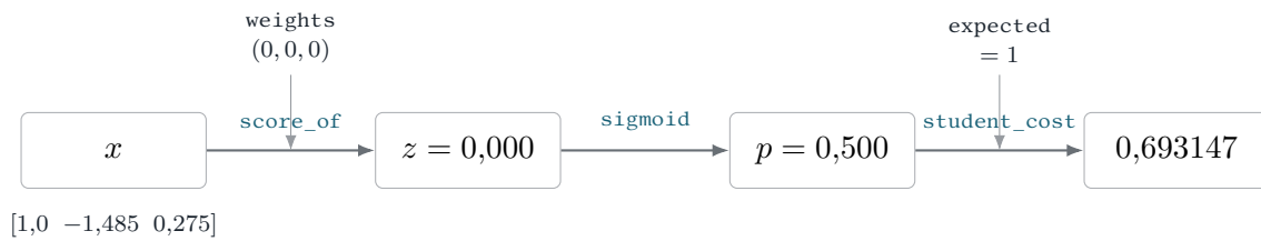
FIGURE 10.4: L'élève 3 traversant les trois fonctions, coefficients nuls. Les coefficients n'interviennent qu'au premier passage, la réponse attendue qu'au dernier.
