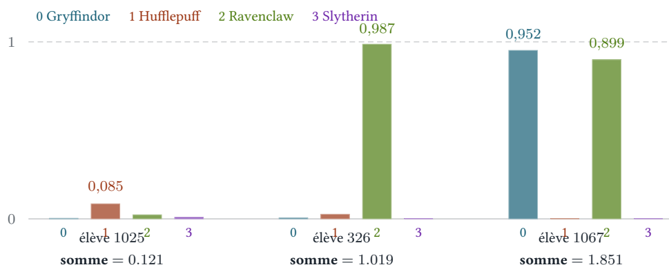
FIGURE 9.3: Quatre sorties sigmoïdées et leur somme, pour trois élèves ; barres numérotées de 0 à 3 dans l'ordre des classes. État M_4 . Sur les 1 600 élèves, la somme excède 1 dans 975 cas.
