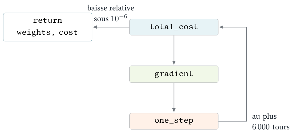
FIGURE 11.3: Le coût est calculé une fois par tour, pour le seul test d'arrêt. Le gradient constitue un second passage sur les 1 600 lignes : une itération en coûte deux.
