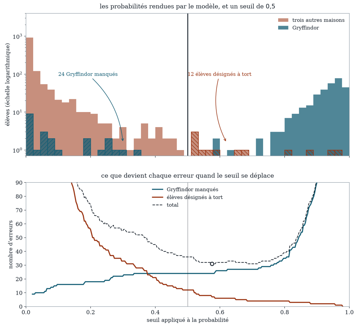
FIGURE 12.5: Probabilités par classe observée, en haut ; hachures : erreurs au seuil 0,5. Nombre d'erreurs selon le seuil, en bas ; minimum cerclé.
