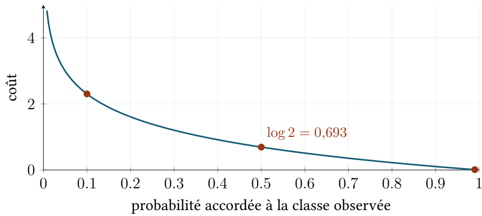
FIGURE E.2: La perte d'une prédiction en fonction de la probabilité que le modèle attribuait à la classe observée. Le point 0,693 correspond à un modèle qui produit 0,5.
