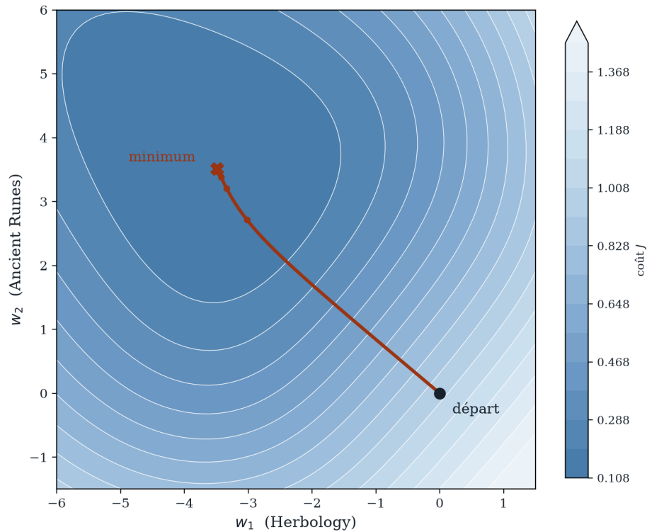
FIGURE I.3: La même surface vue de dessus. Chaque courbe relie les couples de perte égale ; la trajectoire les coupe perpendiculairement. Les points marquent une itération sur vingt-cinq.
