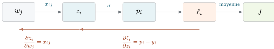
FIGURE F.1: Le coefficient agit sur le coût par cette seule chaîne. Les deux dérivées encadrées se multiplient, et la moyenne donne \partial J / \partial w_j . La propriété \sigma' = \sigma(1 - \sigma) réduit les deux facteurs intermédiaires à p_i - y_i .
