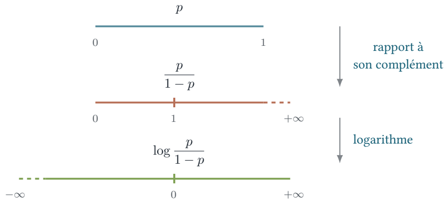
FIGURE C.1: Les trois intervalles. La cote étire ]0, 1[ sur ]0, +\infty[ en envoyant 0,5 sur 1 ; le logarithme envoie ce demi-axe sur \mathbb{R} . La composée est une bijection croissante de ]0, 1[ sur \mathbb{R} , l’une des infinités qui rendent l’égalité avec le score possible (section 2).
