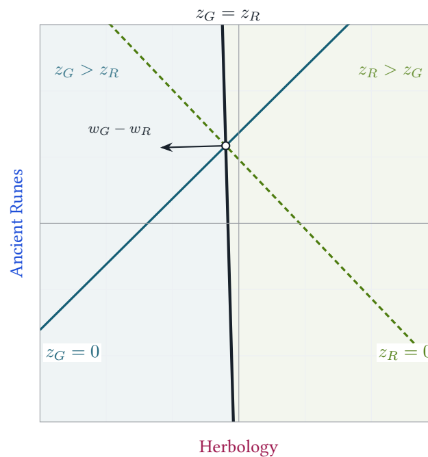
FIGURE K.5: Frontières binaires de Gryffindor (trait plein) et de Ravenclaw (tireté), et limite entre leurs deux régions (trait épais). Cette limite a pour vecteur normal w_G - w_R et passe par l'intersection des deux premières.
