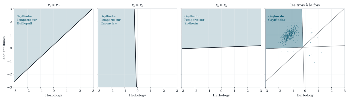
FIGURE K.4: Les trois demi-plans où Gryffindor l'emporte sur chacun de ses rivaux, puis leur intersection. Le dernier panneau porte les observations de cette classe, qui s'y trouvent presque toutes. État du modèle : M_4 .
