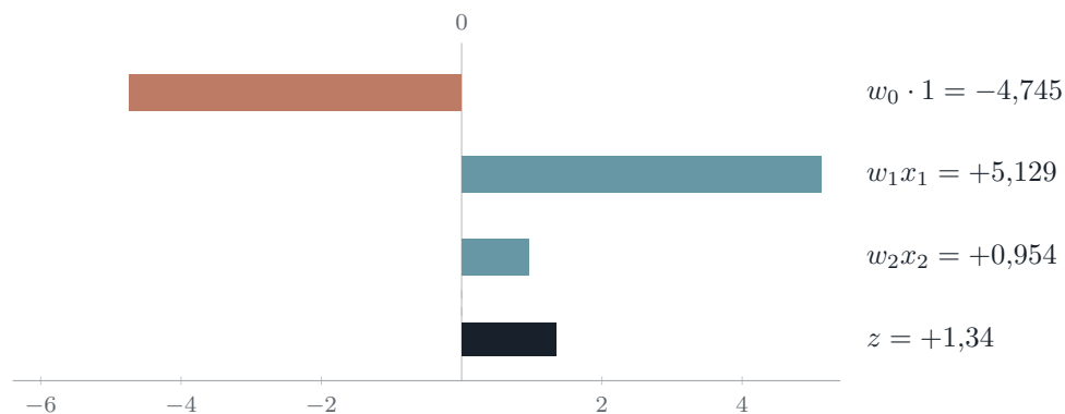
FIGURE 5.2: Les trois termes du score de l'élève 3, à l'échelle : +1,34 pour des contributions individuelles de l'ordre de 5.
