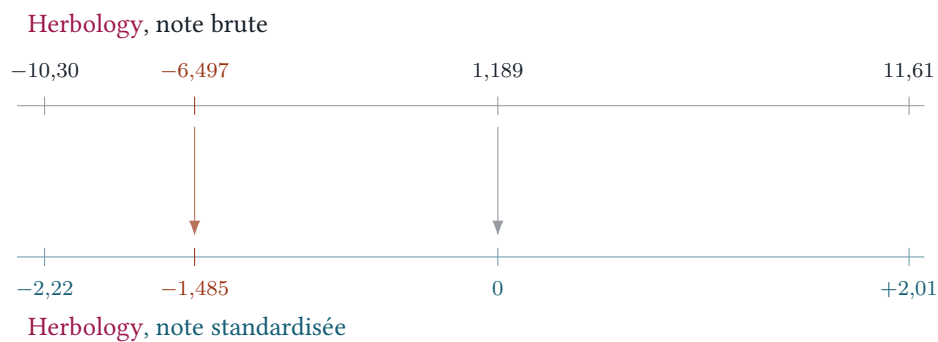
FIGURE 3.1: Sur un seul axe, la transformation est affine croissante : elle déplace l'origine et change l'unité, sans modifier l'ordre des élèves. En rouge, l'élève 3.
