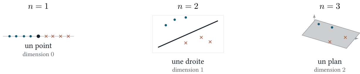
FIGURE K.1: Frontière pour une, deux et trois matières. Disque : classe traitée ; croix : autres classes. Le vecteur normal, |z|/\|w\| et le signe de z conservent leur rôle.
