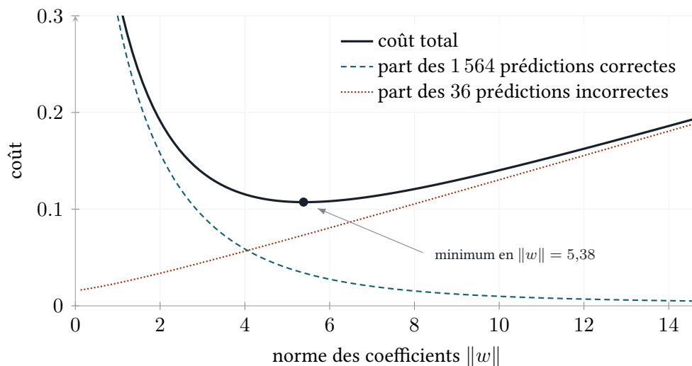
FIGURE H.2: Coût à frontière fixe selon la norme. La part des prédictions correctes décroît; celle des 36 autres croît. Minimum en \|w\| = 5,38 .
