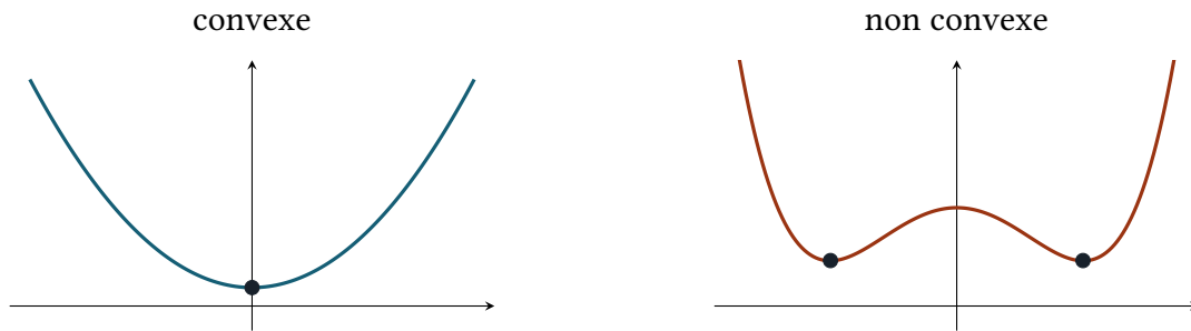
FIGURE G.1: Fonction strictement convexe à minimum unique, à gauche ; fonction à deux minima locaux, à droite. La stricte convexité de la perte logistique demande une condition supplémentaire (section 3).
