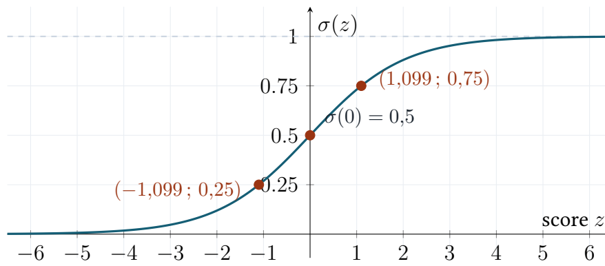
FIGURE C.2: La fonction logistique envoie \mathbb{R} dans l'intervalle ]0, 1[ , sans jamais atteindre les bornes, et passe par 0,5 à l'origine.
