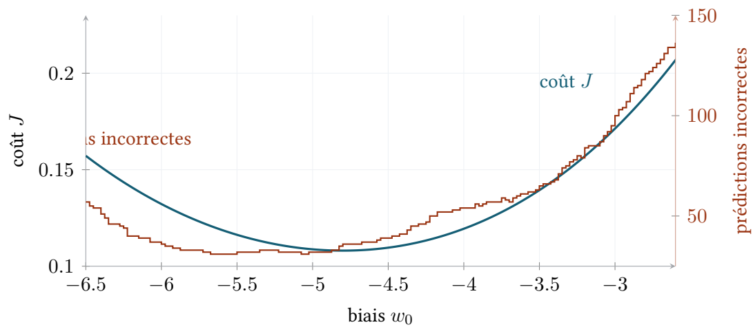
FIGURE 6.2: Coût et nombre d'erreurs selon le biais, à w_1, w_2 fixés. Leurs minima diffèrent : w_0 = -4,80 pour le coût, -5,68 pour les erreurs.
