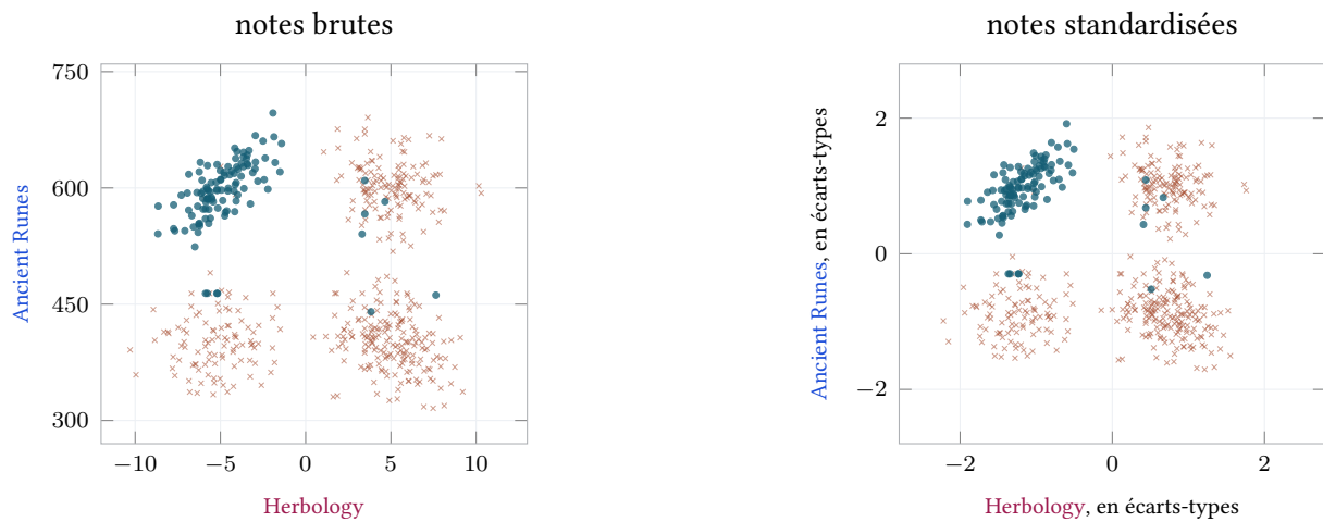
FIGURE 3.2: 534 élèves : Gryffindor en bleu, autres maisons en orangé. Les transformations affines des axes préservent l'ordre et les alignements ; les distances et les angles changent.
