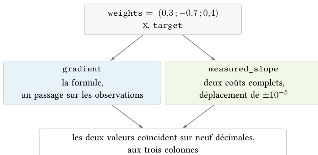
FIGURE 11.1: Deux chemins indépendants vers la même dérivée. Le point d'évaluation est choisi loin de zéro, où plusieurs erreurs classiques rendent zéro des deux côtés.
