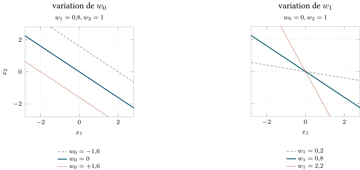
FIGURE K.3: Trait plein commun aux deux panneaux : w = (0 ; 0,8 ; 1) . À gauche, w_0 translate la droite ; à droite, w_1 la fait pivoter autour de l'origine, que w_0 = 0 laisse sur la frontière.
