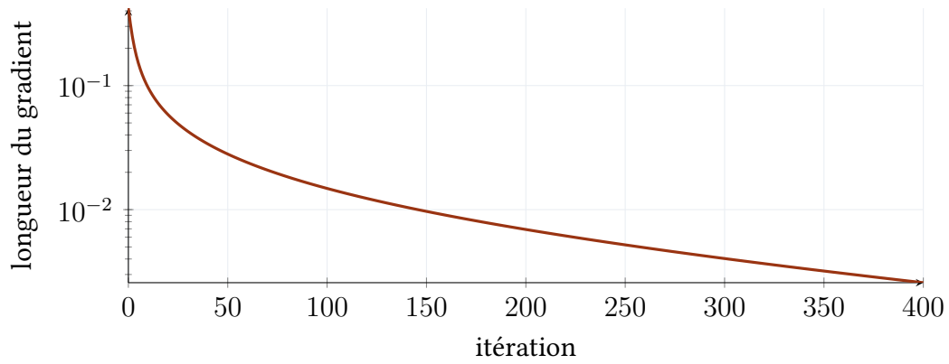
FIGURE I.1: Longueur du gradient en échelle logarithmique, de 0,42 à 0,0026 en 400 itérations. Cette décroissance fournit le critère d'arrêt.
