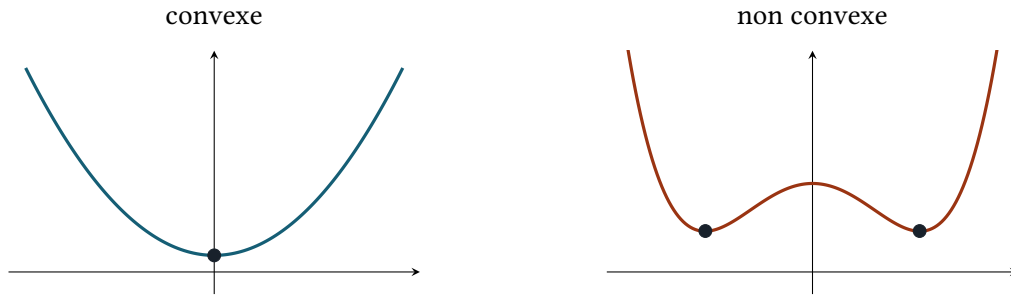
Figure G-A Fonction strictement convexe à minimum unique, à gauche ; fonction à deux minima locaux, à droite. La stricte convexité de la perte logistique demande une condition supplémentaire (section 3).
