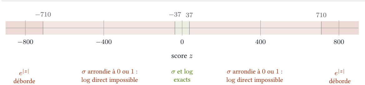
Figure J-A Trois régimes du calcul en double précision. L’écriture directe tient dans la zone centrale ; les formes protégées restent finies sur tout l’axe.
