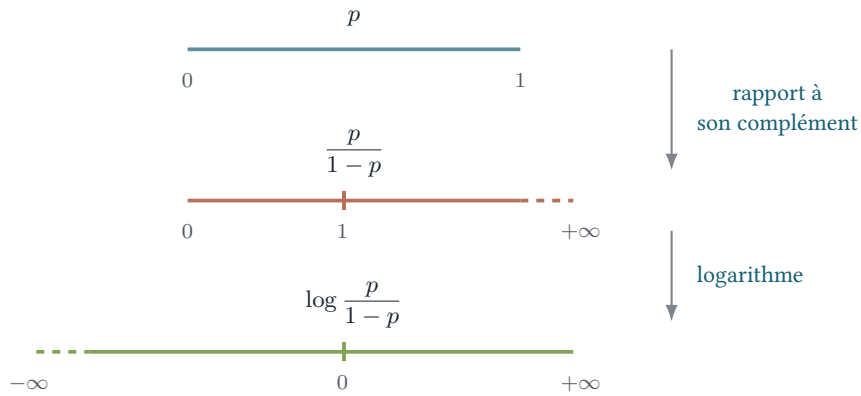
Figure C-A Les trois intervalles. La cote étire ]0, 1[ sur ]0, +\infty[ en envoyant 0,5 sur 1 ; le logarithme envoie ce demi-axe sur \mathbb{R} . La composée est une bijection croissante de ]0, 1[ sur \mathbb{R} , l'une des infinités qui rendent l'égalité avec le score possible (section 2).
