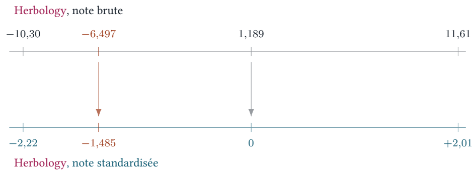
Figure 1-A Sur un seul axe, la transformation est affine croissante : elle déplace l'origine et change l'unité, sans modifier l'ordre des élèves. En rouge, l'élève 3.
