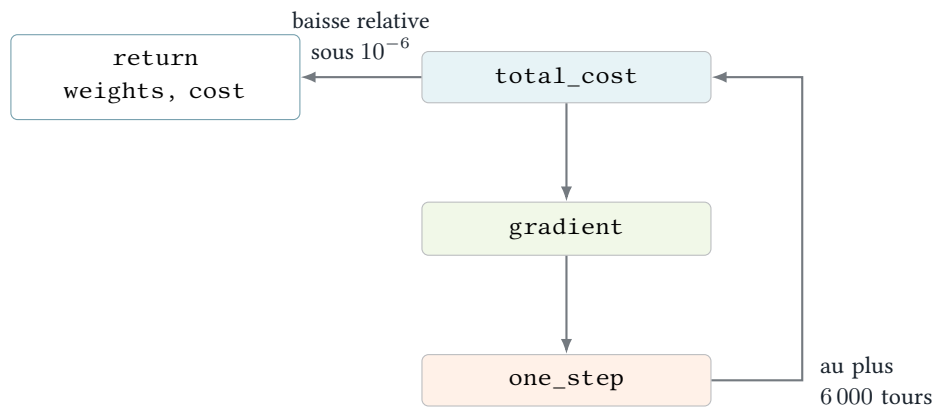
Figure 9-C Le coût est calculé une fois par tour, pour le seul test d'arrêt. Le gradient constitue un second passage sur les 1 600 lignes : une itération en coûte deux.
