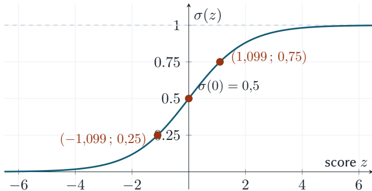
Figure 12 – La fonction logistique envoie \mathbb{R} dans l'intervalle ]0, 1[ , sans jamais atteindre les bornes, et passe par 0,5 à l'origine.
