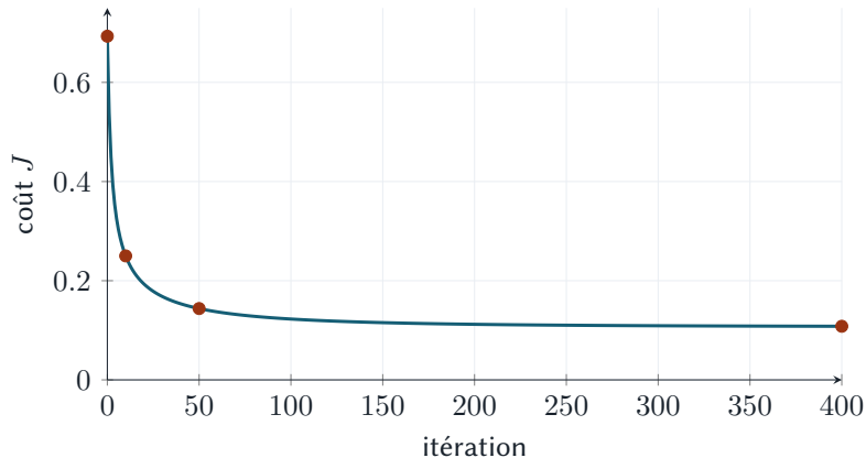
Figure 23 – Perte moyenne aux itérations 0, 10, 50 et 400. Les dix premiers tours couvrent 75,7 % de la baisse totale; les 350 derniers, 6 %.
