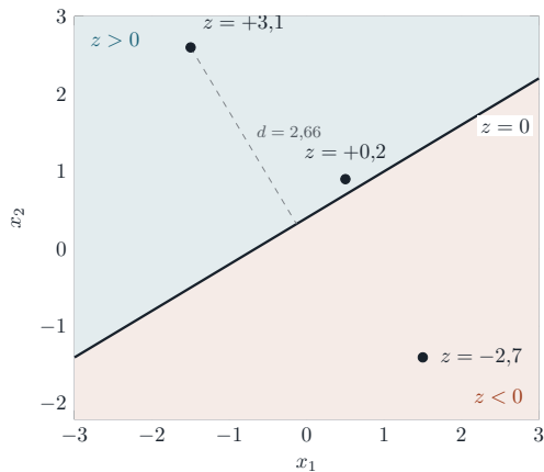
Figure 10 – Frontière pour w = (-0,4; -0,6; 1) . Les distances orthogonales des points de scores +3,1 et +0,2 valent respectivement 2,66 et 0,17 .
