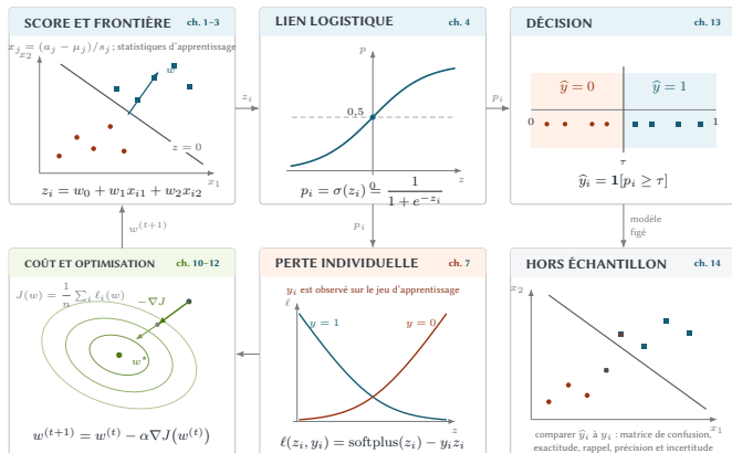
Figure 1 – Vue d'ensemble du modèle. La rangée supérieure transforme une observation en classe prédite pour des coefficients fixés. La rangée inférieure relie l'étiquette observée à la perte, à l'optimisation des coefficients et au contrôle sur un jeu tenu hors de l'ajustement.
