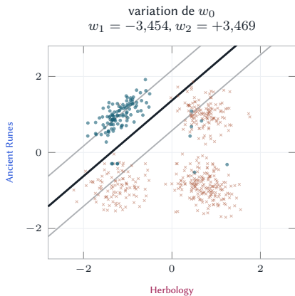
Figure 31 – Variation isolée du biais, à gauche : translation. Variation isolée de w_1 , à droite : rotation et modification de la pente de la sigmoïde.
