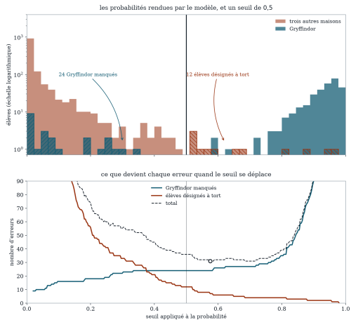
Figure 40 – Probabilités par classe observée, en haut; hachures : erreurs au seuil 0,5. Nombre d'erreurs selon le seuil, en bas; minimum circled.
