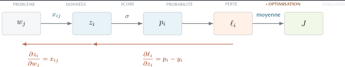
Figure 22 – Le coefficient agit sur le coût par cette seule chaîne. Les deux dérivées encadrées se multiplient, et la moyenne donne \partial J / \partial w_j . La propriété \sigma' = \sigma(1 - \sigma) réduit les deux facteurs intermédiaires à p_i - y_i .
