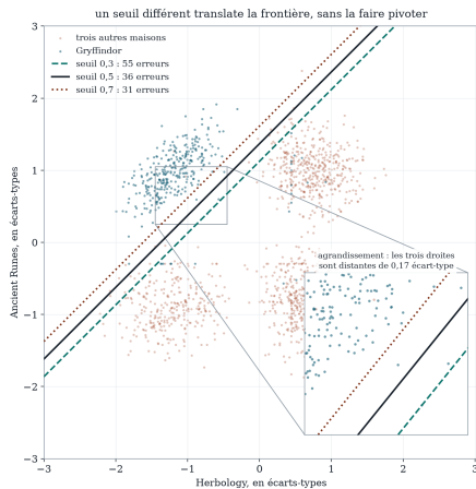
Figure 41 – Nuage standardisé et droites des seuils 0,3, 0,5 et 0,7 : même direction, biais décalés. L'agrandissement porte les observations qui changent de réponse d'une droite à l'autre.
