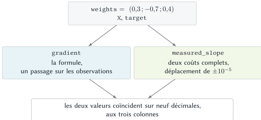
Figure 28 – Deux chemins indépendants vers la même dérivée. Le point d'évaluation est choisi loin de zéro, où plusieurs erreurs classiques rendent zéro des deux côtés.
