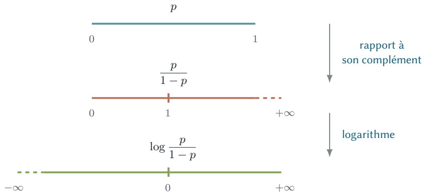
Figure 11 – Les trois intervalles. La cote étire ]0, 1[ sur ]0, +\infty[ en envoyant 0,5 sur 1 ; le logarithme envoie ce demi-axe sur \mathbb{R} . La composée est une bijection croissante de ]0, 1[ sur \mathbb{R} , l’une des infinités qui rendent l’égalité avec le score possible (section 2).
