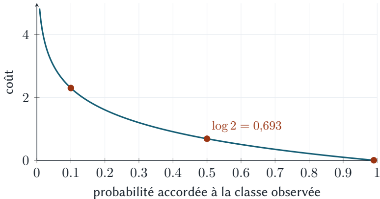
Figure 18 – La perte d’une prédiction en fonction de la probabilité que le modèle attribuait à la classe observée. Le point 0,693 correspond à un modèle qui produit 0,5.
