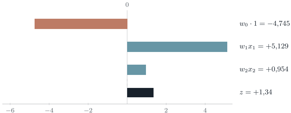
Figure 14 – Les trois termes du score de l'élève 3, à l'échelle : +1,34 pour des contributions individuelles de l'ordre de 5.
