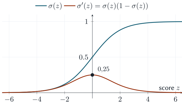
Figure 15 – La dérivée atteint son maximum, 0,25, en z = 0 , et tend vers zéro dès que la probabilité approche 0 ou 1.
