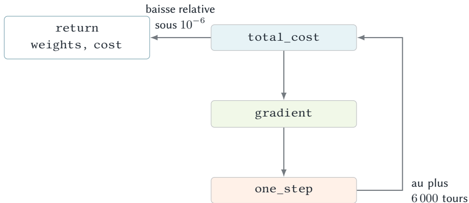
Figure 30 – Le coût est calculé une fois par tour, pour le seul test d'arrêt. Le gradient constitue un second passage sur les 1 600 lignes : une itération en coûte deux.
