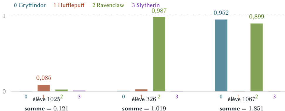
Figure 35 – Quatre sorties sigmoïdées et leur somme, pour trois élèves; barres numérotées de 0 à 3 dans l'ordre des classes. État M_4 . Sur les 1 600 élèves, la somme excède 1 dans 975 cas.
