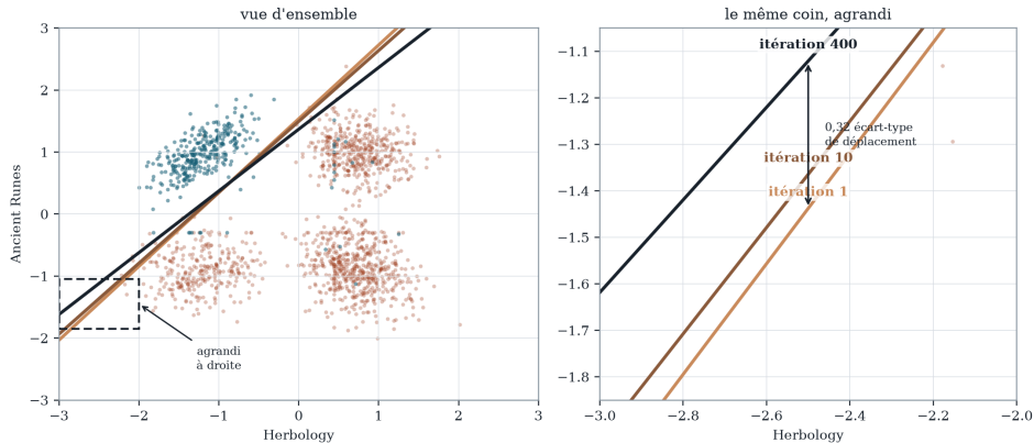
Figure 24 – Frontière aux itérations 1, 10 et 400; le rectangle agrandi sépare les trois droites. Elles pivotent autour d'un point central du nuage, pour un déplacement total d'un tiers d'écart-type.
