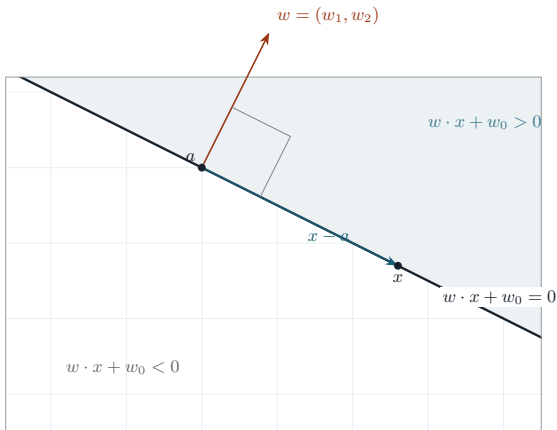
Figure 9 – La droite est l'ensemble des points x tels que x - a soit perpendiculaire à w . Le vecteur w pointe vers le demi-plan où l'expression w \cdot x + w_0 est positive.
