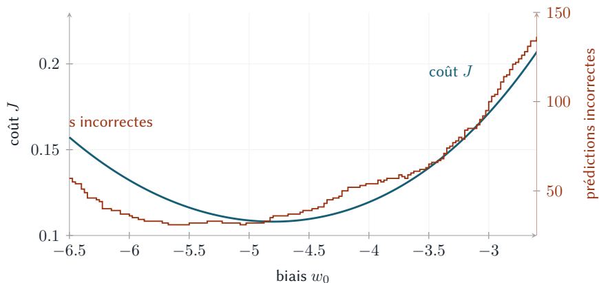
Figure 19 – Coût et nombre d’erreurs selon le biais, à w_1, w_2 fixés. Leurs minima diffèrent : w_0 = -4,80 pour le coût, -5,68 pour les erreurs.
