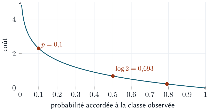
Figure 16 – Perte associée à une prédiction. Elle vaut \log 2 en 0,5, tend vers zéro à droite et croît sans borne à gauche.
