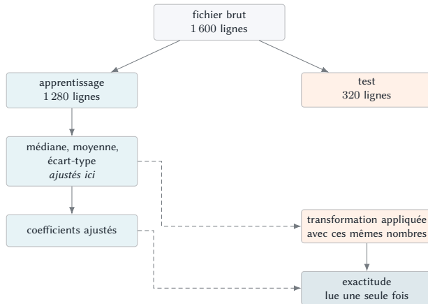
Figure 37 – Les statistiques de préparation sont des paramètres ajustés au même titre que les coefficients. Les flèches en pointillé transportent des nombres figés, jamais un nouvel ajustement.
