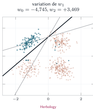
Figure 31 – Variation isolée du biais, à gauche : translation. Variation isolée de w_1 , à droite : rotation et modification de la pente de la sigmoïde.
