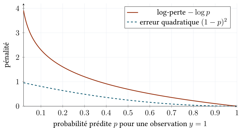
FIGURE 4.2 – Comparaison pour y = 1 . Les deux pertes sont minimales en p = 1 , mais la log-perte pénalise beaucoup plus fortement une probabilité presque nulle attribuée à l'événement réellement observé. Elle découle en outre directement de la vraisemblance de Bernoulli.
