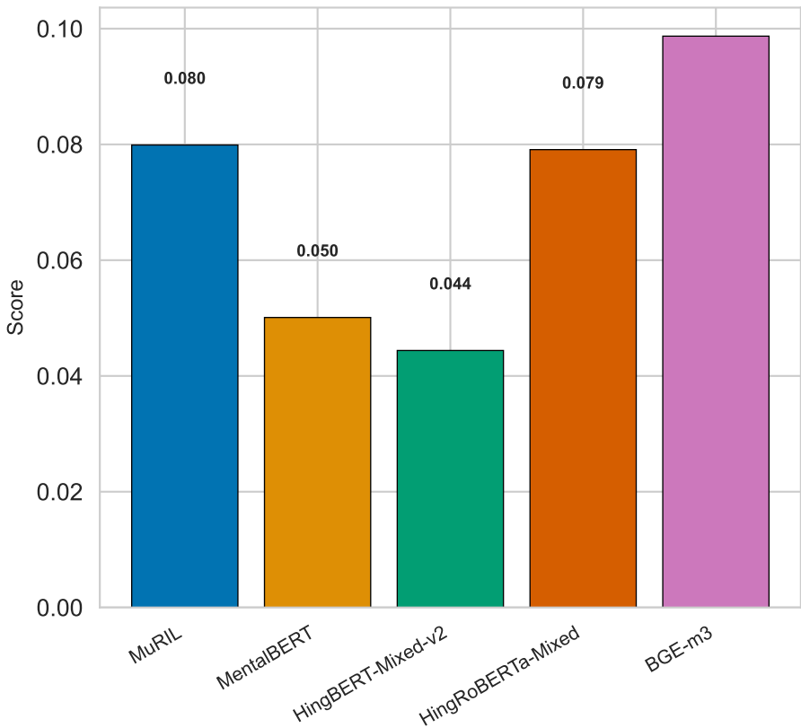
Retrieval P@10
