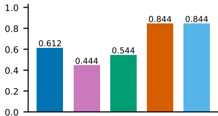
Retrieval P@10
