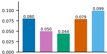
Coherence c_{npmi}
