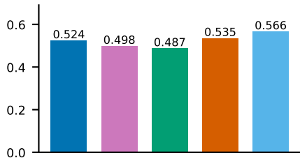
Coherence c_v
