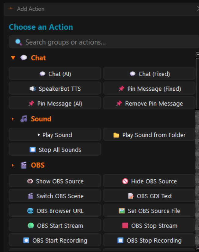
Das Fenster „Choose an Action“ mit allen Aktionsgruppen
