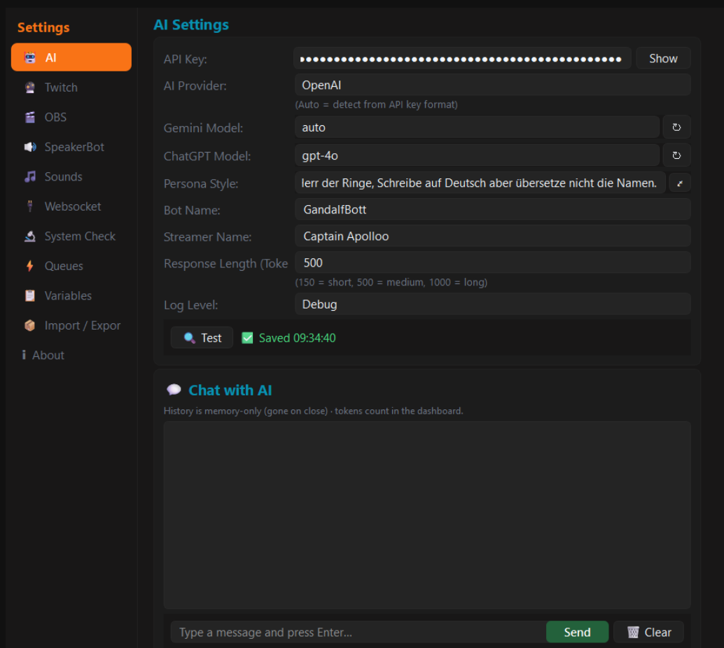
Die AI Settings mit dem Chatfenster darunter
