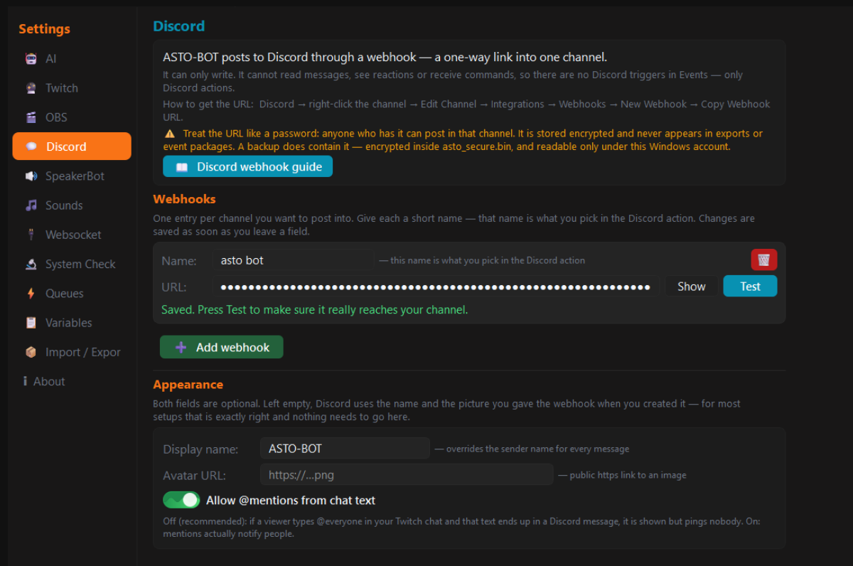
Der Discord-Bereich in den Settings mit einem angelegten Webhook
