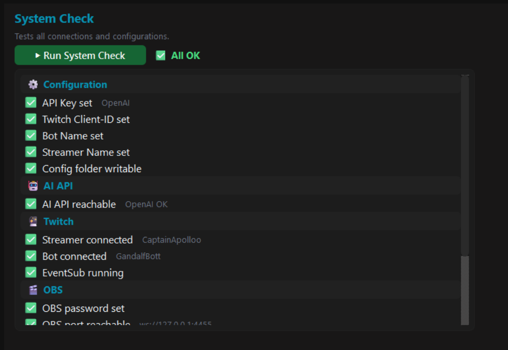
Der System Check prüft Konfiguration, KI, Twitch und OBS
