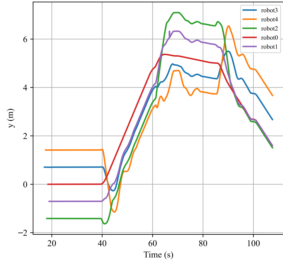
Y Evolution
