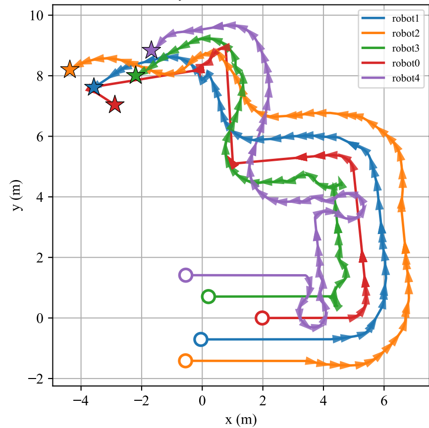
Trayectoria de los robots
