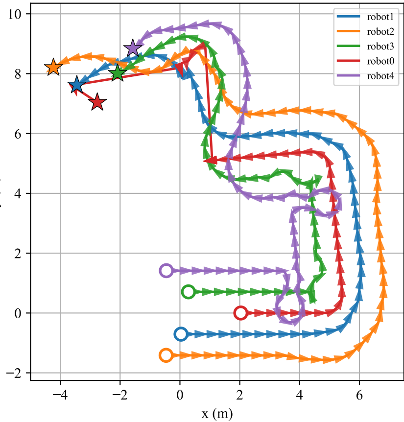
Robot trajectories
