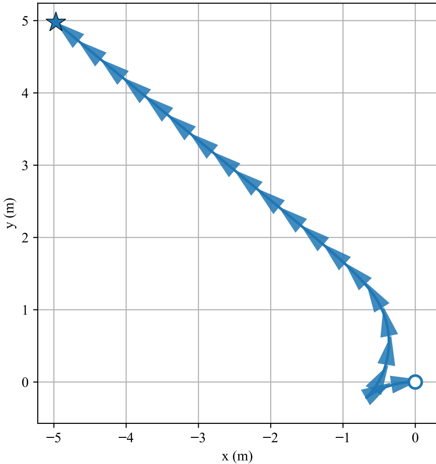
Robot trajectory
