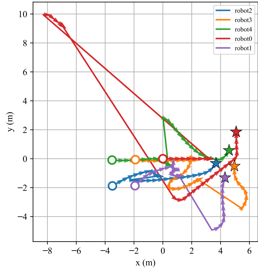
Robot trajectories
