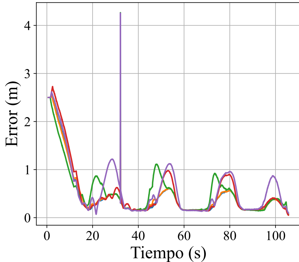
Evolución del error de formación
