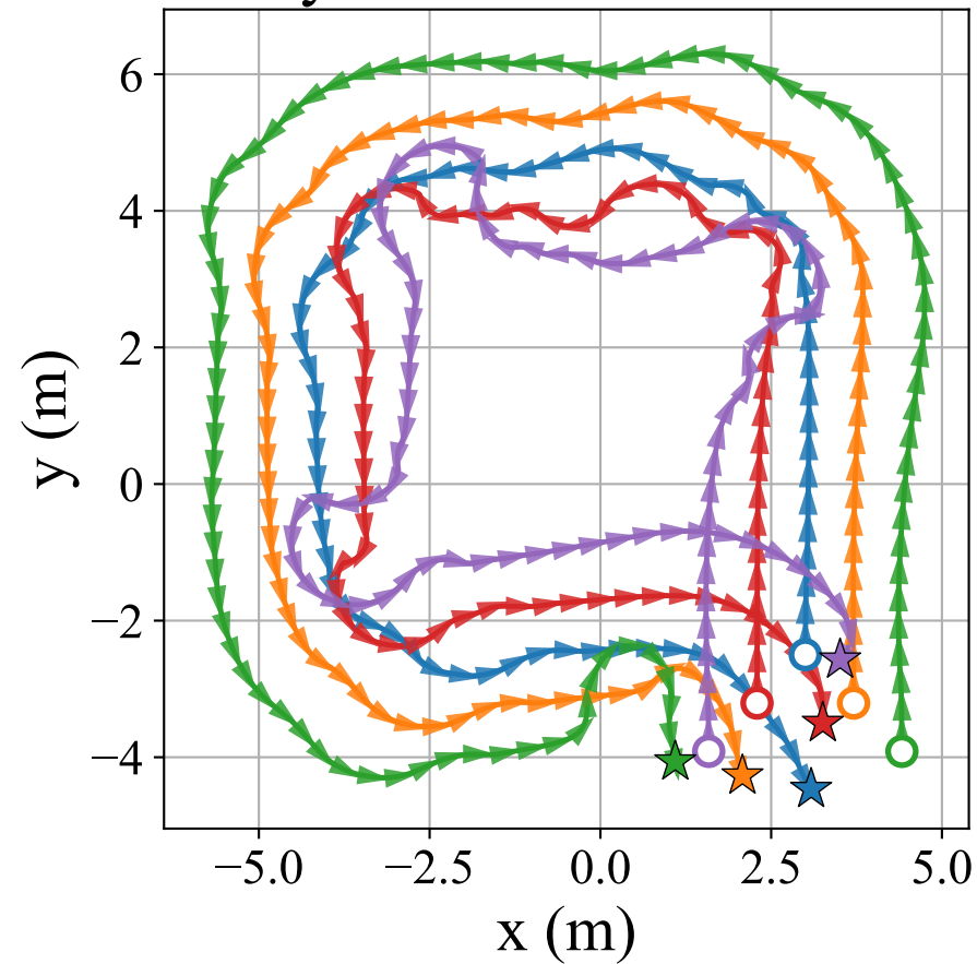
Trayectorias de los robots
