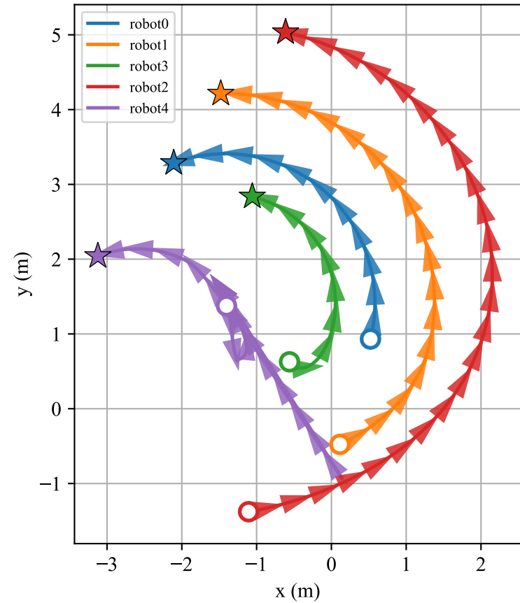
Robot trajectories
