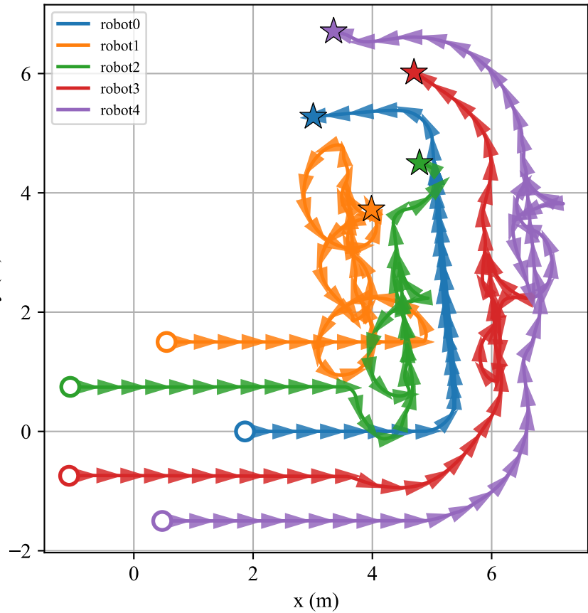
Robot trajectories
