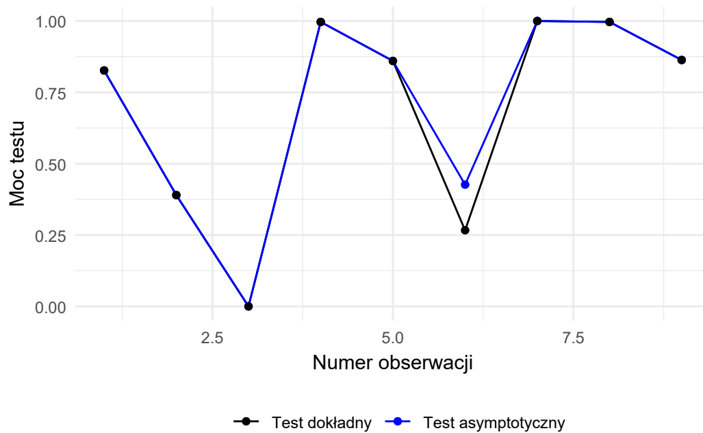
Rysunek 10: Porównanie mocy testów dokładnego i asymptotycznego
