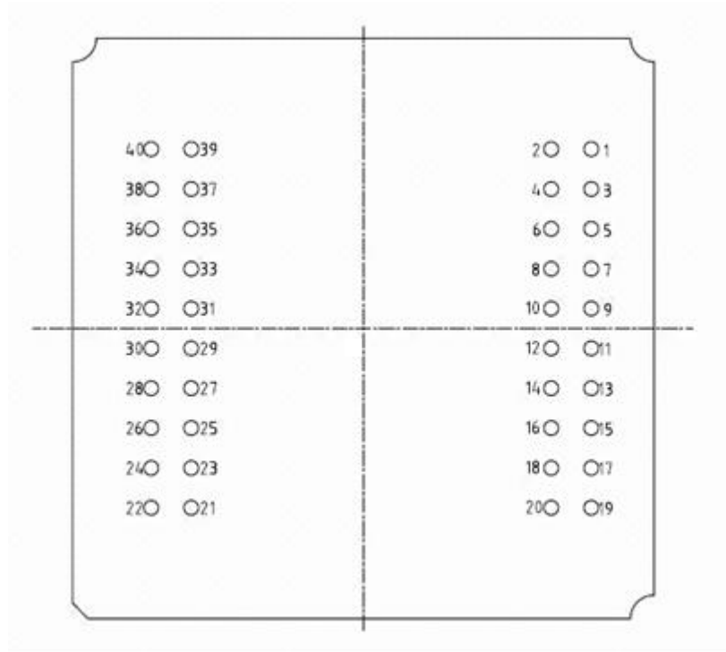
图1-1 I/O管脚示意图
