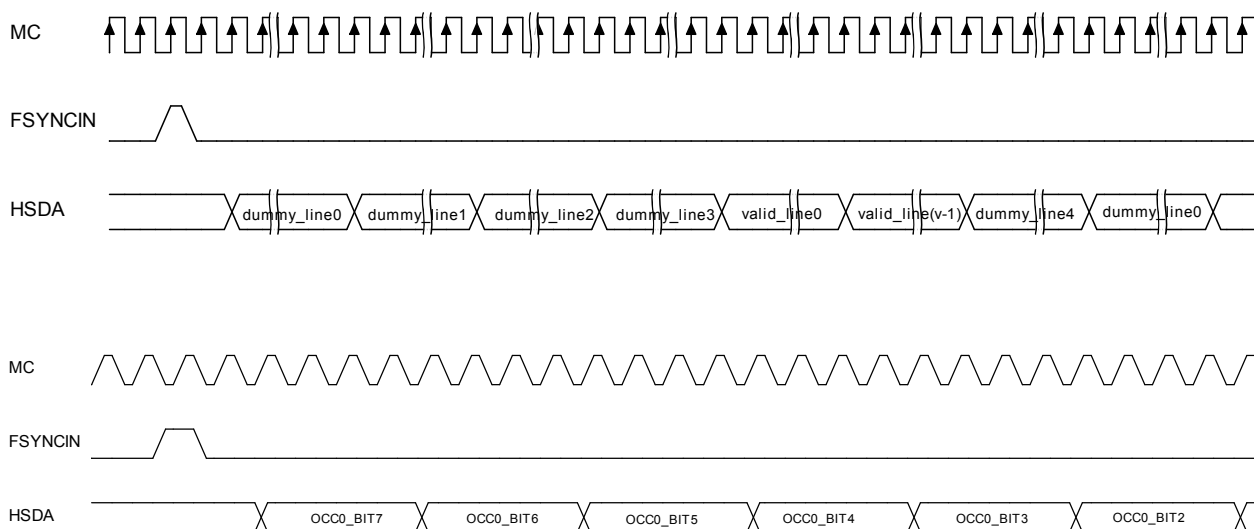
图5-6 时钟与数字输入时序图
