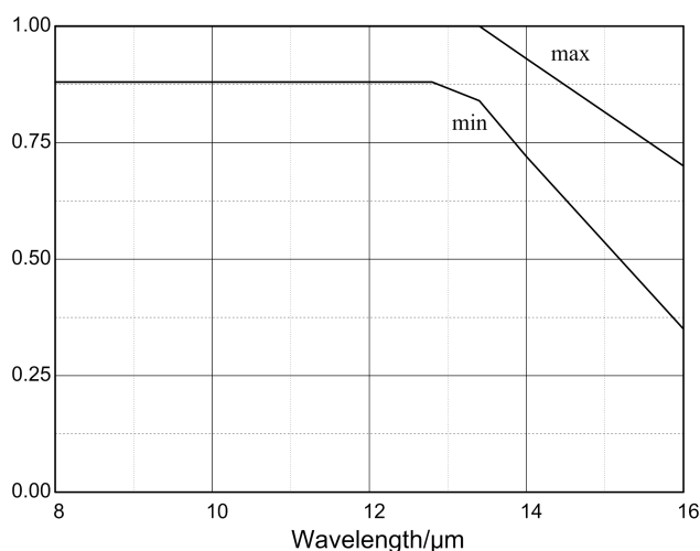
图2-1 归一化的GST412C0的光谱响应
