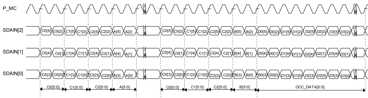
图5-4 时钟与数字输入时序图
