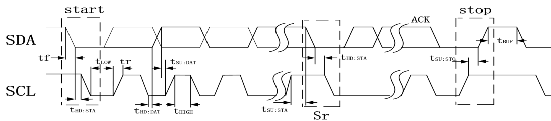
图5-1 IIC时序
