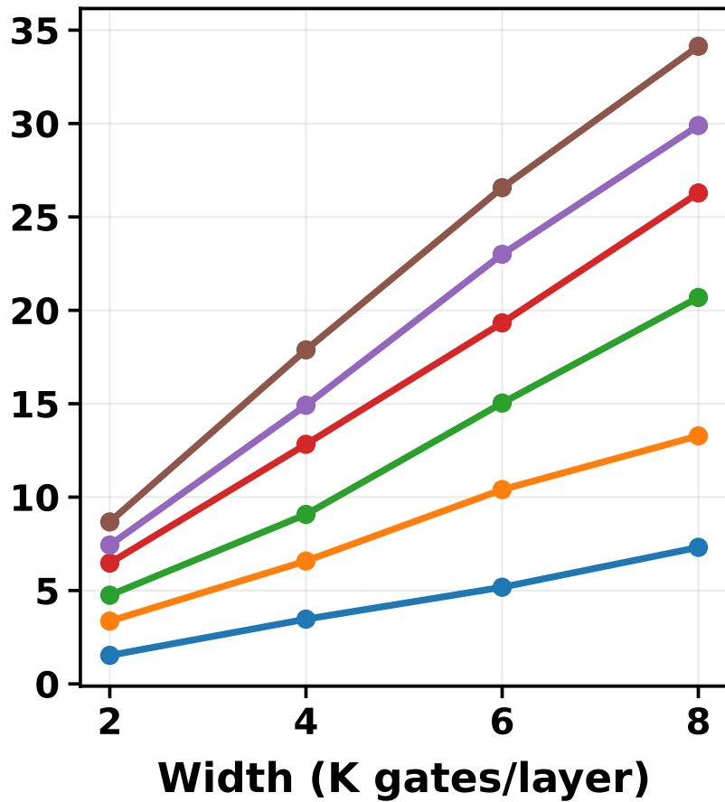
MNIST
