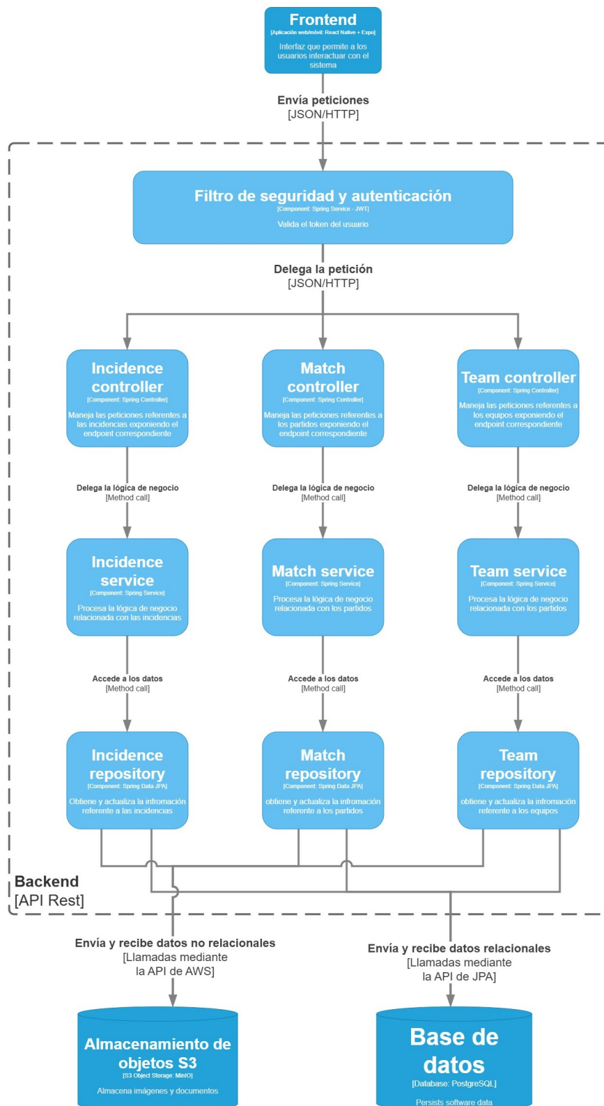
Figura G.3: Modelo C4 nivel 3: arquitectura de tres capas
