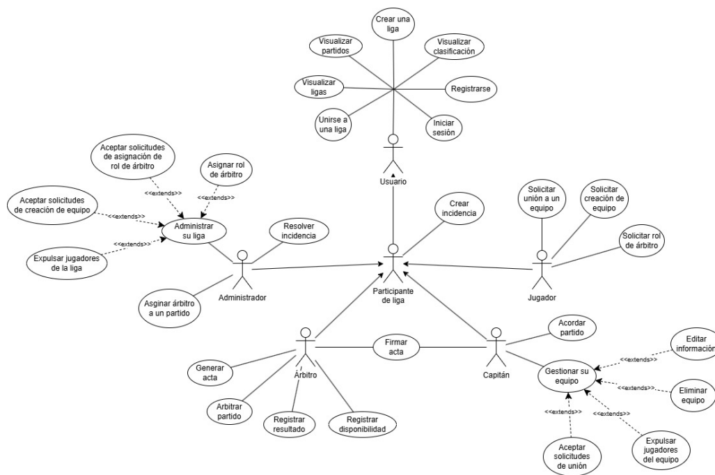
Figura D.1: Diagrama de casos de uso
