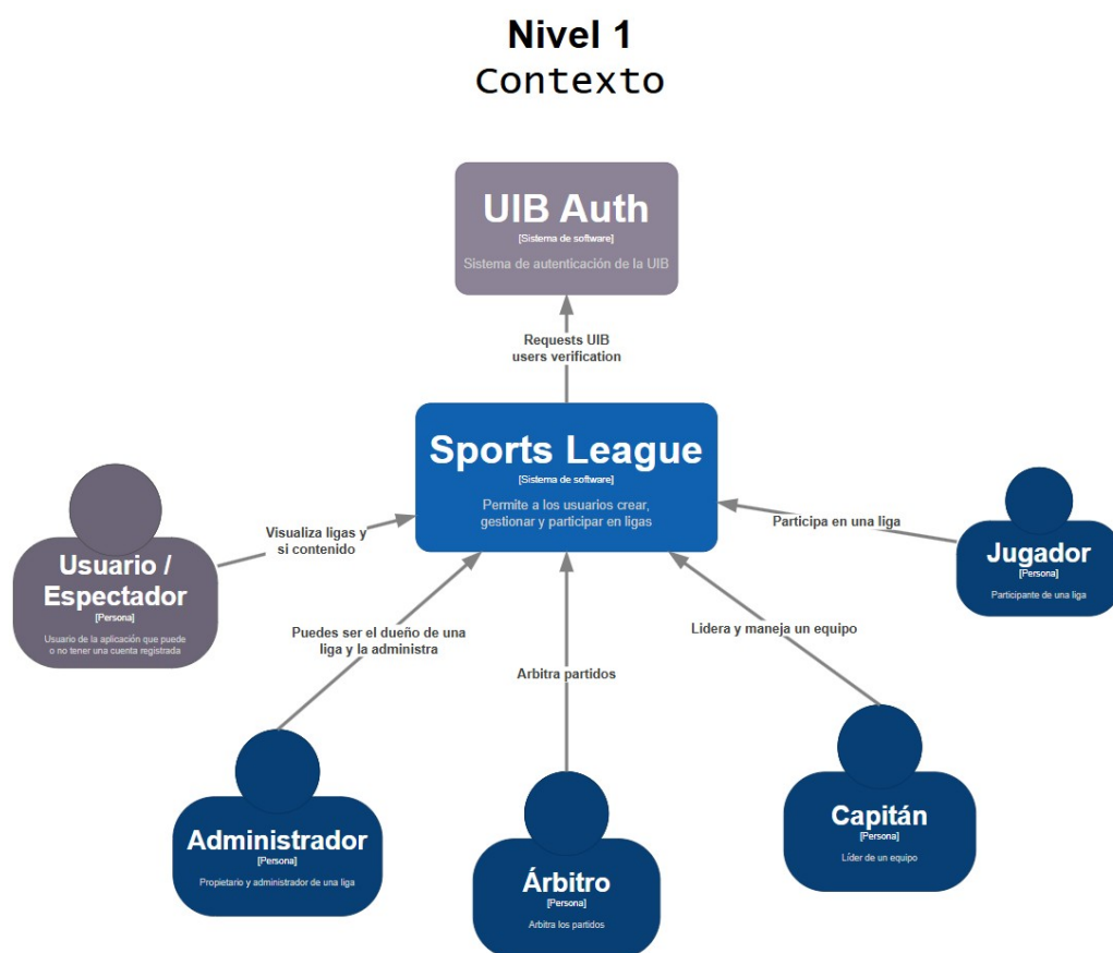
Figura G.1: Modelo C4 nivel 1
