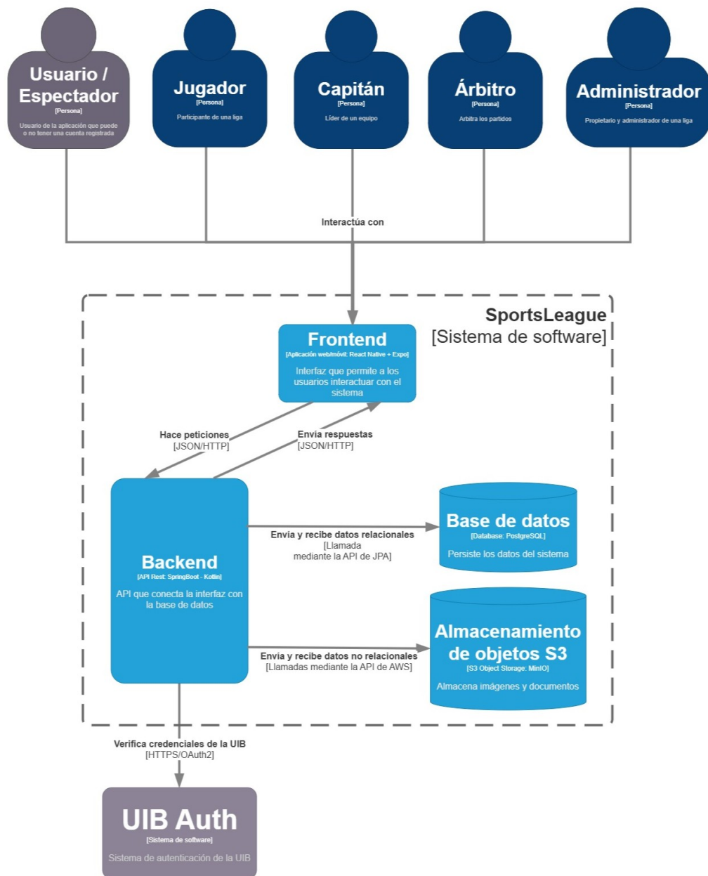
Figura G.2: Modelo C4 nivel 2
