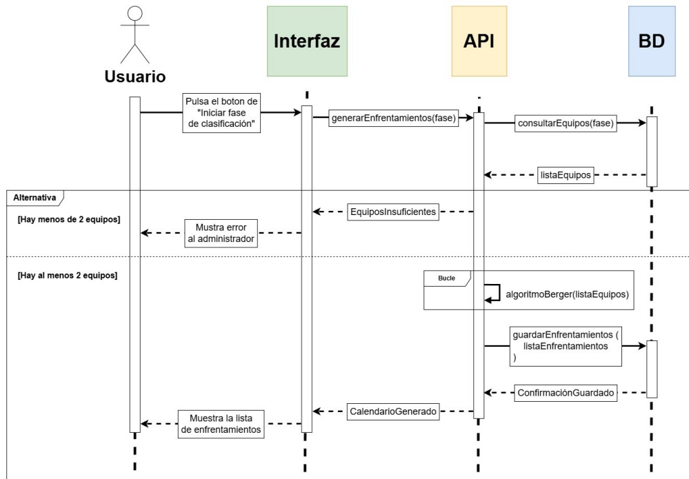
Figura G.6: Diagrama Usuario-Sistema para el caso de uso de Crear Enfrentamientos
