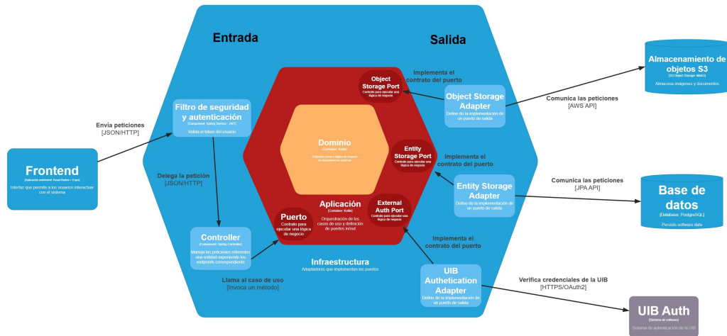
Figura G.4: Modelo C4 nivel 3: arquitectura hexagonal
