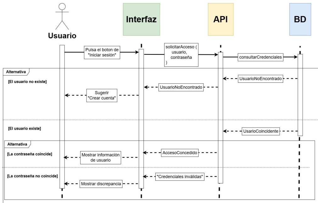
Figura G.5: Diagrama Usuario-Sistema para el caso de uso de Iniciar Sesión
