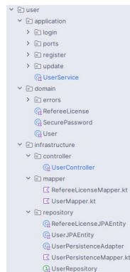
(a) Ejemplo de módulo con arquitectura hexagonal
