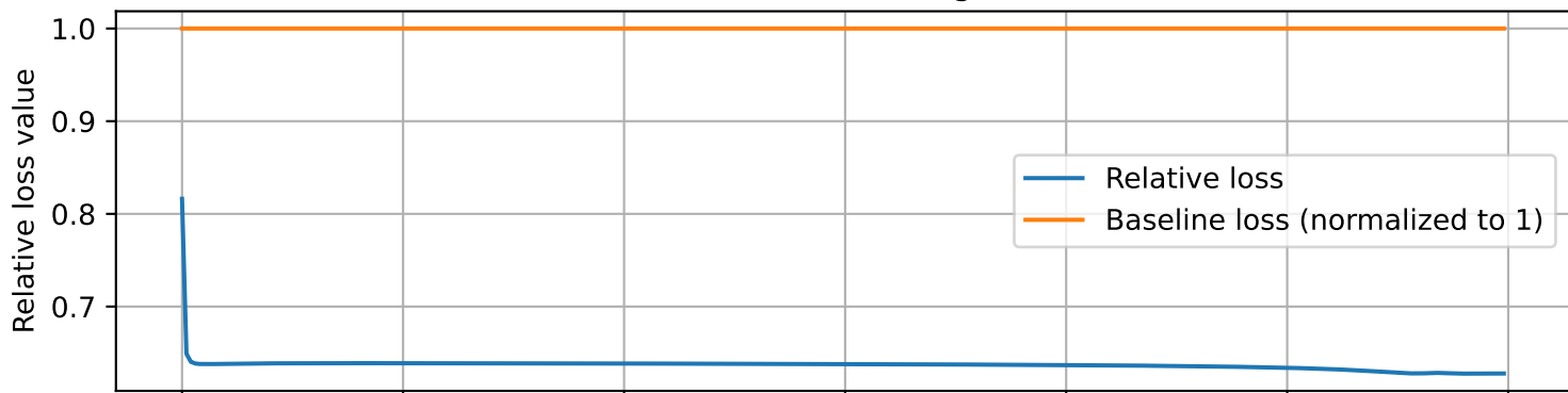
Parameters convergence
