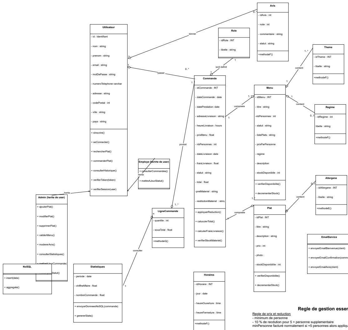
DIAGRAMME DE CLASSE UML
