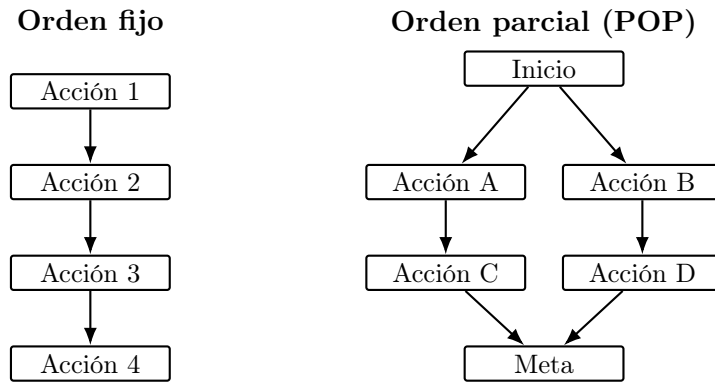
Figura 7.7: Orden fijo vs. orden parcial: en el plan de orden fijo cada acción depende rígidamente de la anterior; en POP, las acciones A/B (y C/D) son mutuamente independientes y solo se ordenan respecto a lo que sí exigen sus dependencias reales, dejando margen para ejecutarlas en cualquier orden entre sí o en paralelo.
