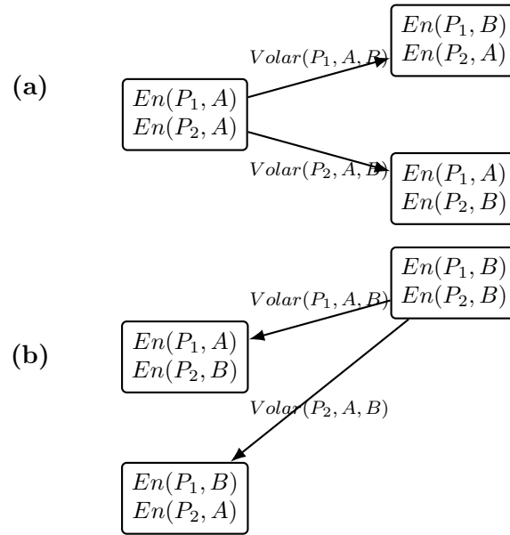
Figura 7.5: (a) Búsqueda hacia adelante: desde el estado inicial, cada avión disponible genera una rama distinta al aplicar Volar . (b) Búsqueda hacia atrás: desde una meta con ambos aviones en B , cada regresión sobre Volar genera un estado predecesor distinto, según cuál avión se supone que ya voló.
