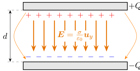
Figura 3.1: Schema in sezione di un condensatore a facce piane parallele. Nella regione centrale il campo elettrico \mathbf{E} è uniforme e perpendicolare alle armature. Ai margini si notano i cosiddetti “effetti di bordo”, trascurabili se d \ll \sqrt{A} .
