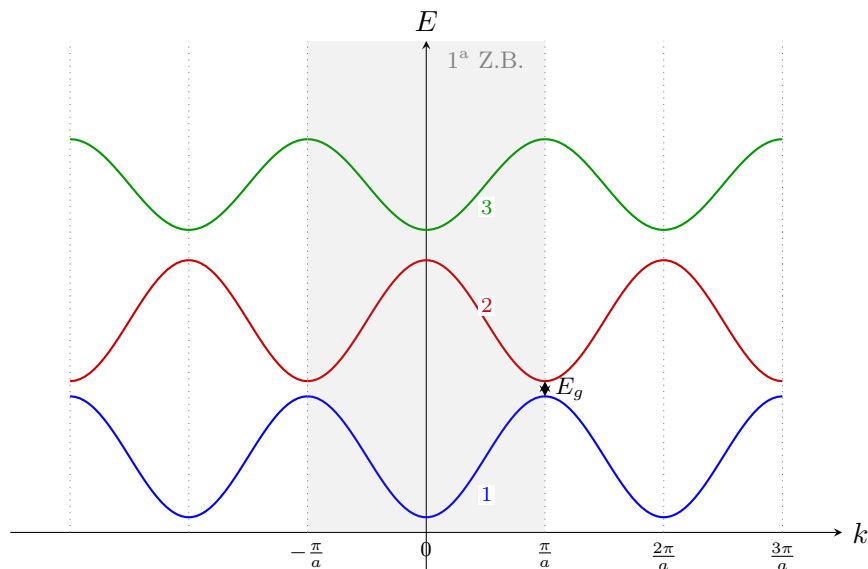
Figura 16.4: Schema a zone ripetute. Poiché l'energia è una funzione periodica nel reticolo reciproco ( E(k) = E(k + G) ), è possibile rappresentare l'intera struttura a bande ripetendo la prima zona di Brillouin.
