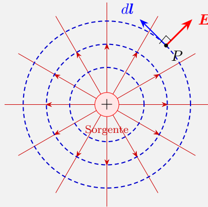
Figura 1.4: Rappresentazione di campo generato da carica puntiforme: linee di campo (rosse) e superfici equipotenziiali (blu). Si nota l'ortogonalità locale in P .
