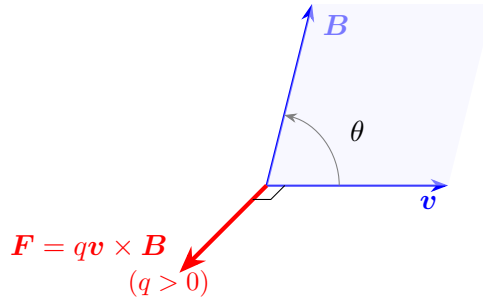
Figura 4.2: Rappresentazione vettoriale della forza di Lorentz. La forza \mathbf{F} è sempre perpendicolare al piano individuato dai vettori velocità \mathbf{v} e campo magnetico \mathbf{B} , secondo la regola della mano destra (per q > 0 ).
