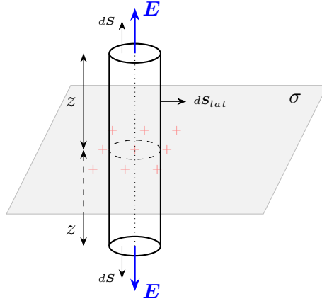
Figura 2.1: Superficie gaussiana cilindrica che attraversa un piano infinito carico. Il flusso attraverso la superficie laterale è nullo perché il campo è radente alla superficie.
