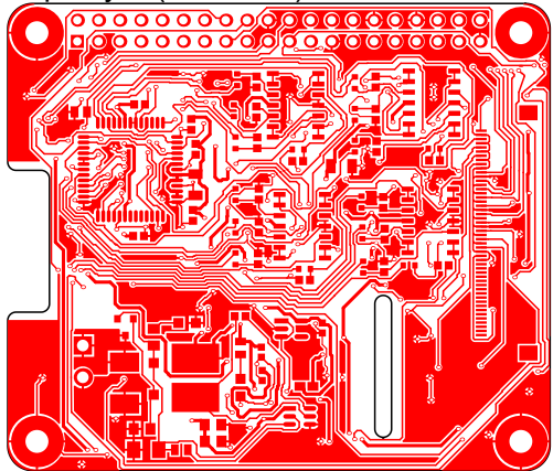
Top Layer (Scale 1:1)
