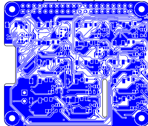
Bottom Layer (Scale 1:1)
