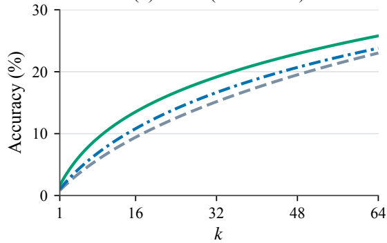
(b) AIME (2024–2026)
