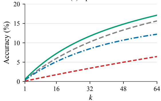
(c) Apex2025
