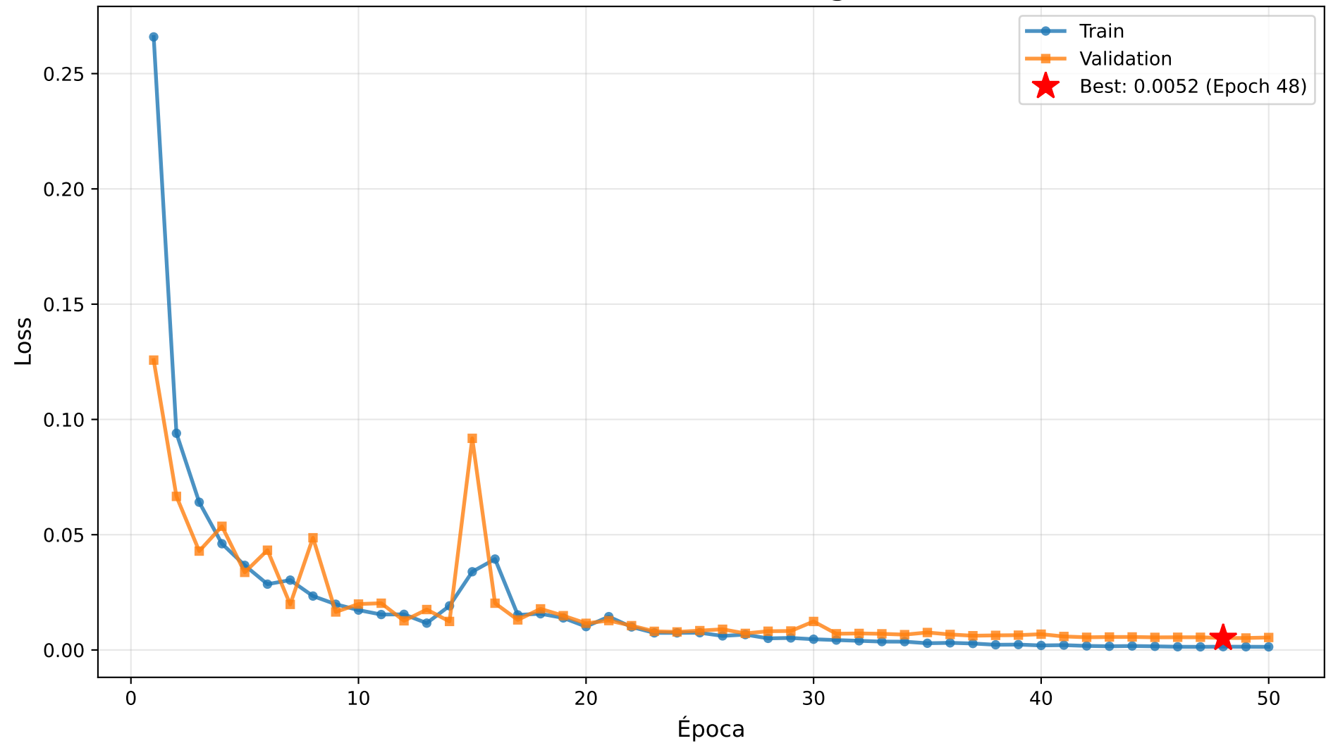
Pérdida de RPN BBox Regression
