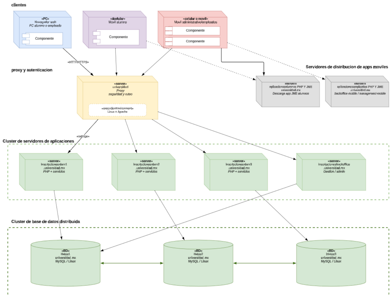
Diagrama de Despliegue
