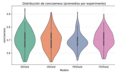
(d) Conciseness
