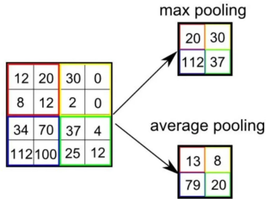
Figura 2.7: En la figura se ve ve cómo se aplica max pooling y average pooling a una entrada. Como las ventanas tienen tamaño 2 \times 2 se dice que se aplica pooling 2 \times 2 . Imagen extraída de https://saturncloud.io/blog/a-comprehensive-guide-to-convolutional-neural-networks-the-eli5-way/ .
