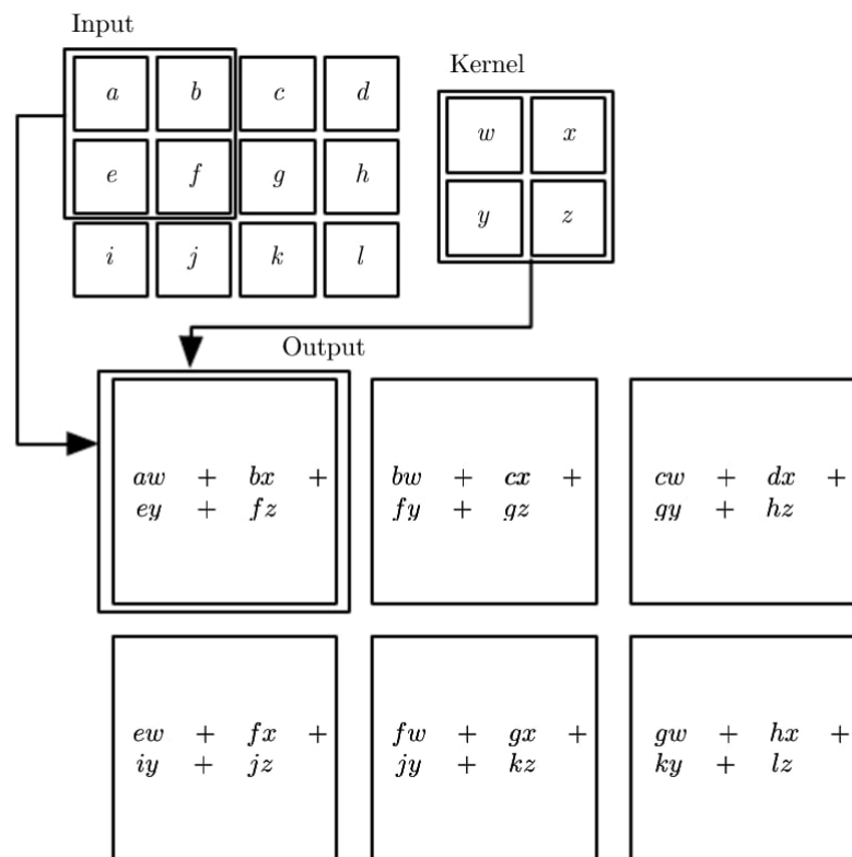
Figura 2.5.: En esta imagen se puede ver un ejemplo de una convolución aplicada a una entrada de dimensiones 3 \times 4 por un kernel de dimensiones 2 \times 2 . Se puede ver que la salida tiene tamaño 2 \times 3 . Notablemente se puede ver que al contrario que en la definición de la operación de convolución dada, aquí no se le da la vuelta al kernel, como suele ocurrir en la práctica. Imagen extraída de (Goodfellow y cols., 2016).
