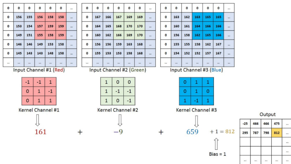
Figura 2.6.: Aquí se puede ver un ejemplo de una convolución aplicada a una entrada con 3 canales, uno por cada color primario. Se ve cómo el kernel ahora tiene 3 canales también. Imagen extraída de https://saturncloud.io/blog/a-comprehensive-guide-to-convolutional-neural-networks-the-eli5-way/ .
