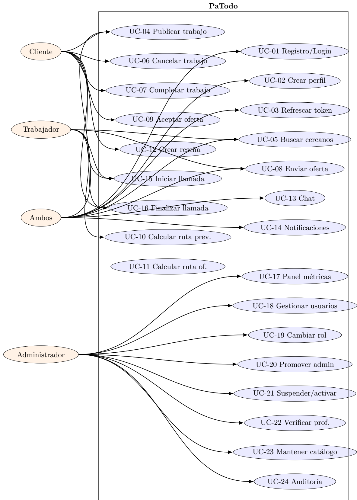
Diagrama de casos de uso del sistema.
