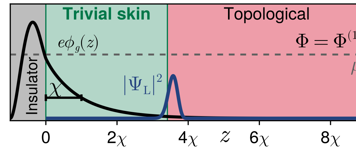
True MZM
