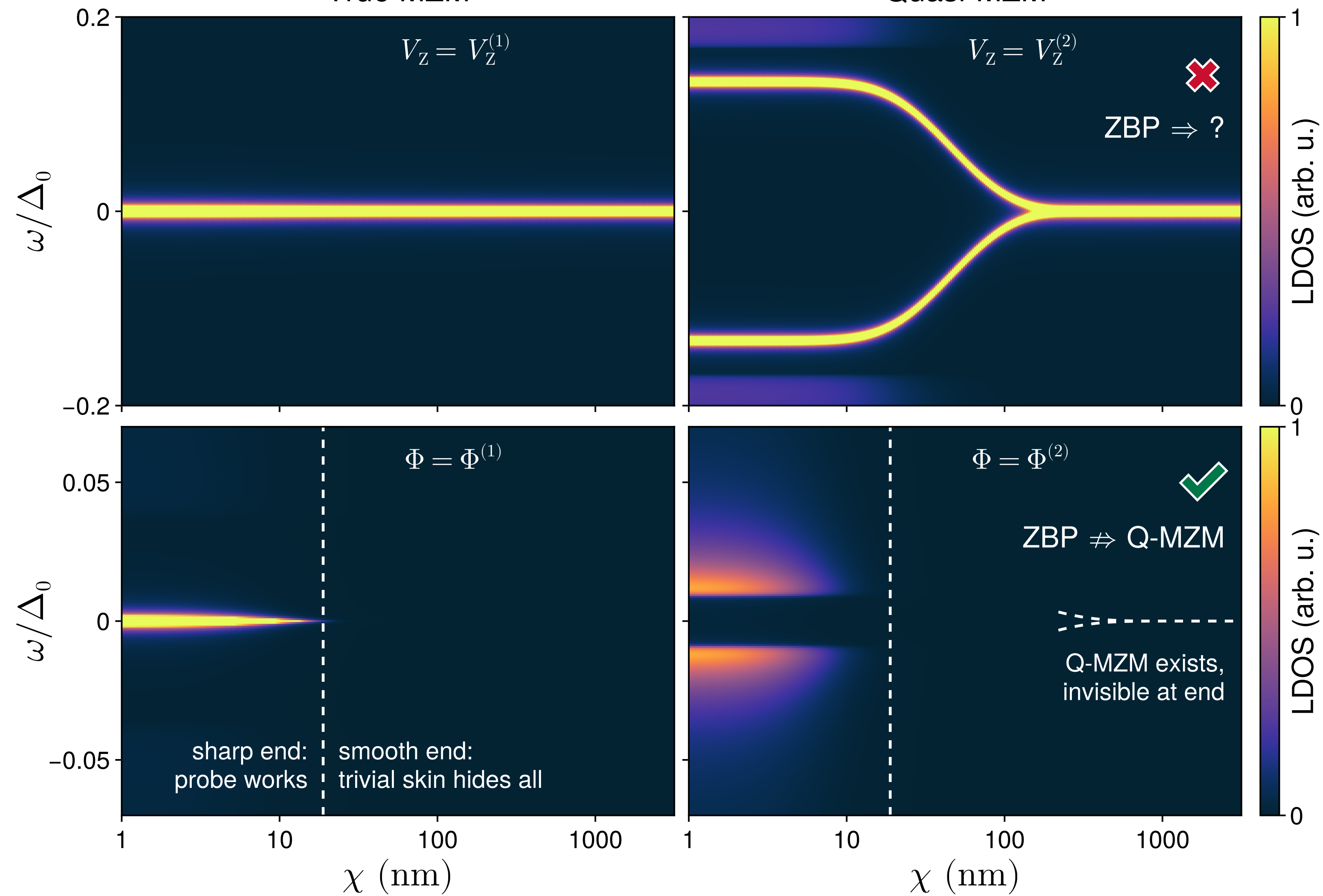
True MZM
