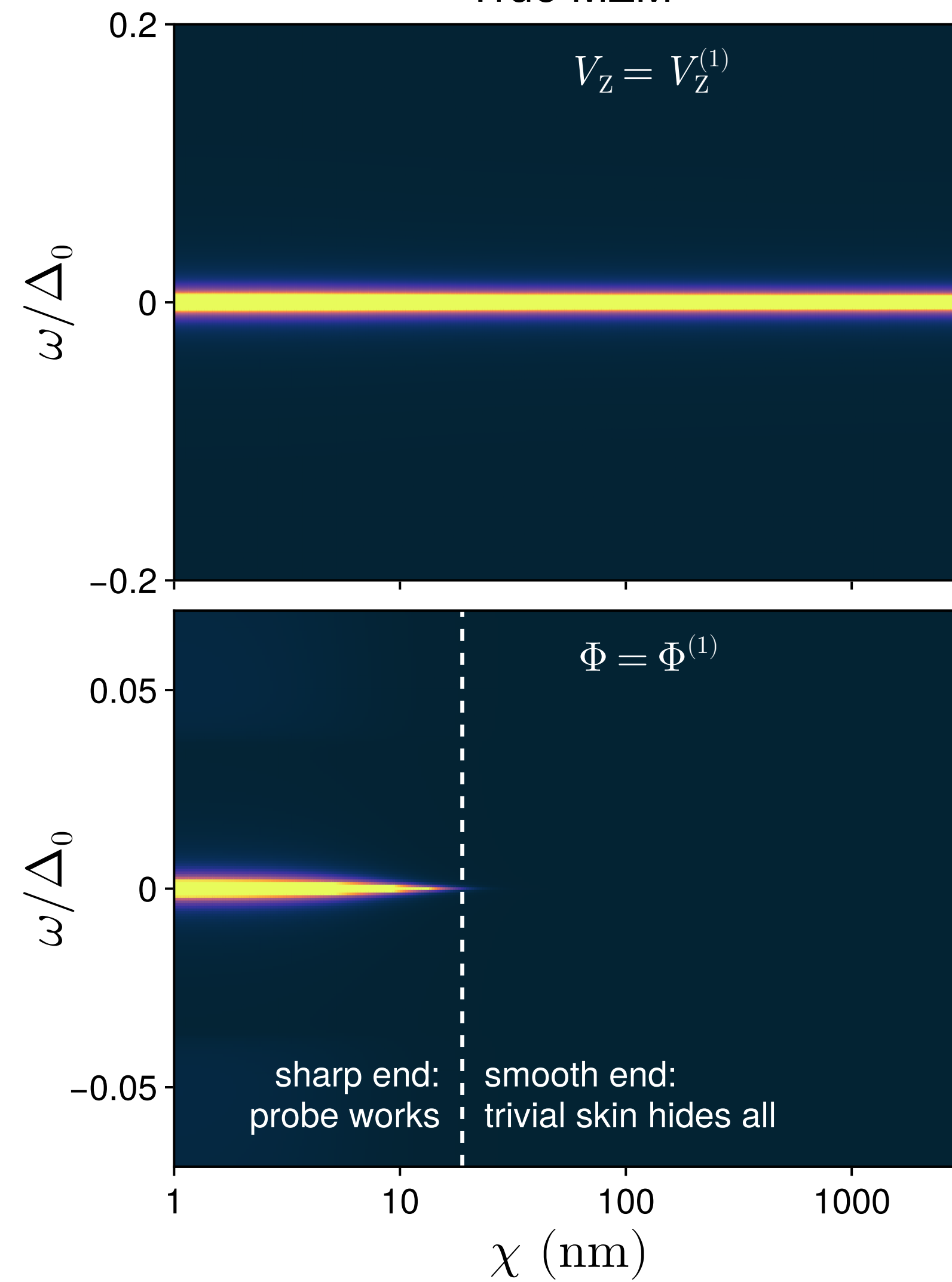
True MZM
