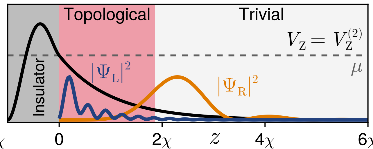
Quasi-MZM
