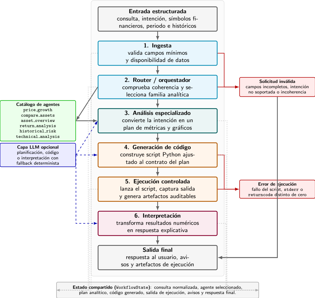
Grafo de orquestación del flujo multiagente
