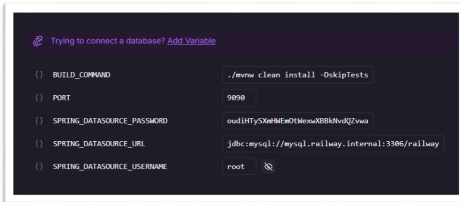
Figura 5 - Variables de Entorno del Back del Railway
