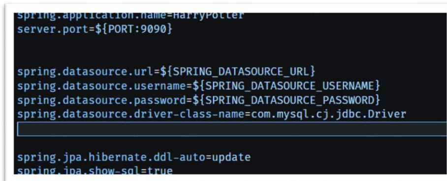
Figura 6 - Archivo Propertires de Springboot
