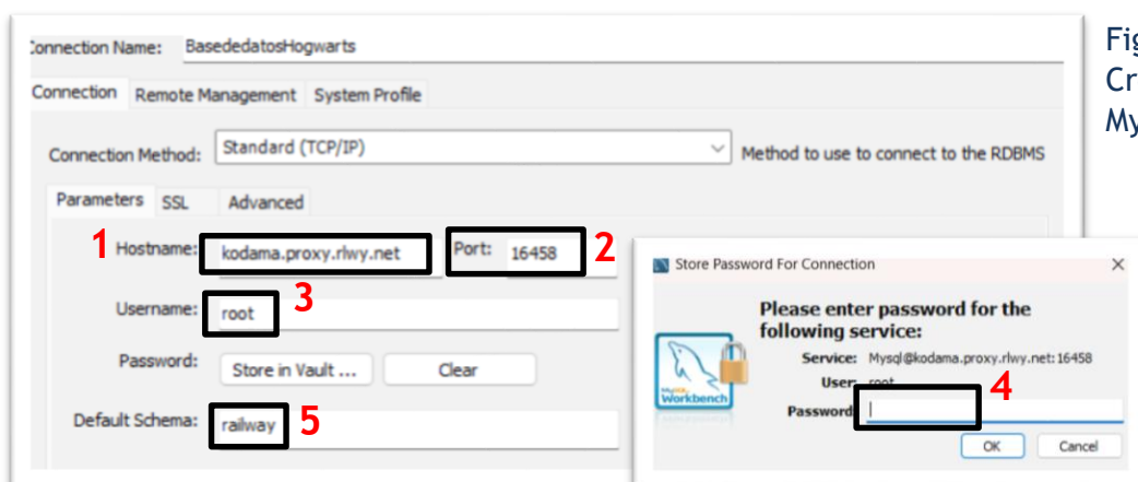
Figura 4 - Conectores del servicio de MySQL de Railway
