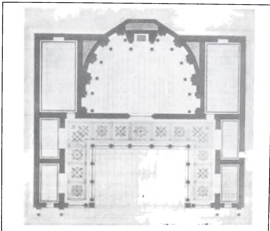
FIGURA 7.6. Plano de la biblioteca de Timgad. Siglo III d.C.
