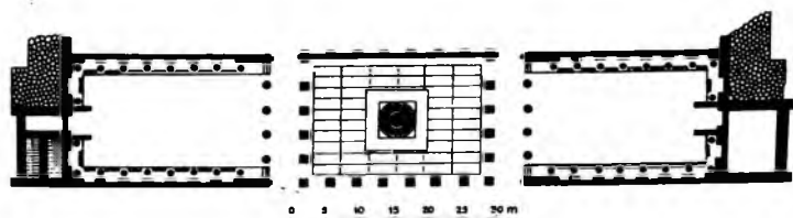
FIGURA 6.3. Plano de las bibliotecas gemelas del Foro de Trajano, Roma. Están una frente a otra con la Columna de Trajano y el pórtico en medio.
