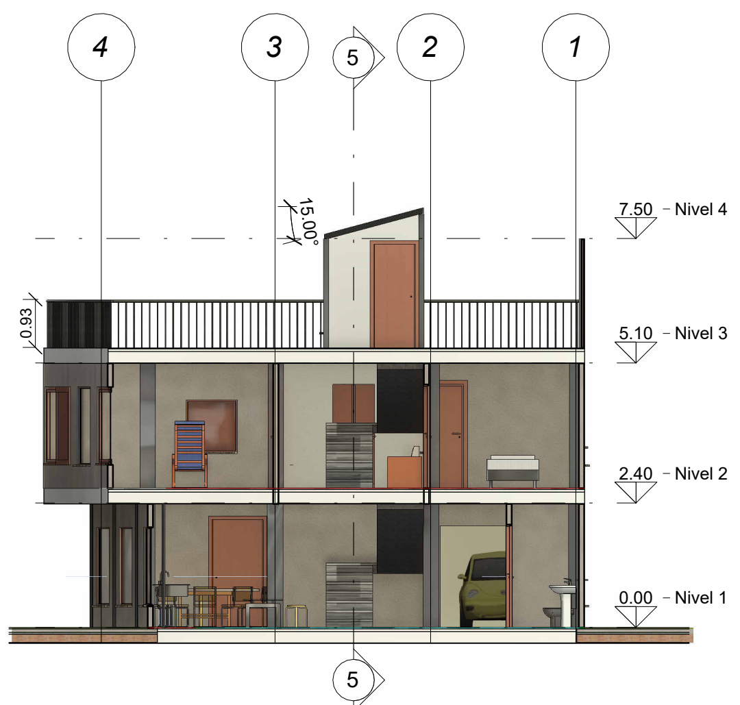
6 Sección 2 A101 1:100
