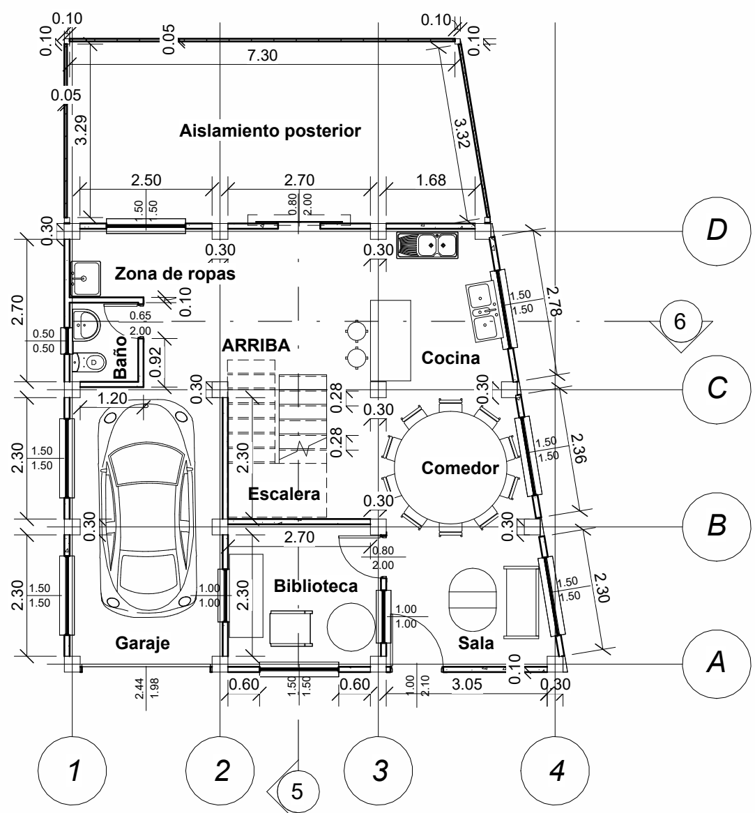
2 Nivel 1 A101 1:100
