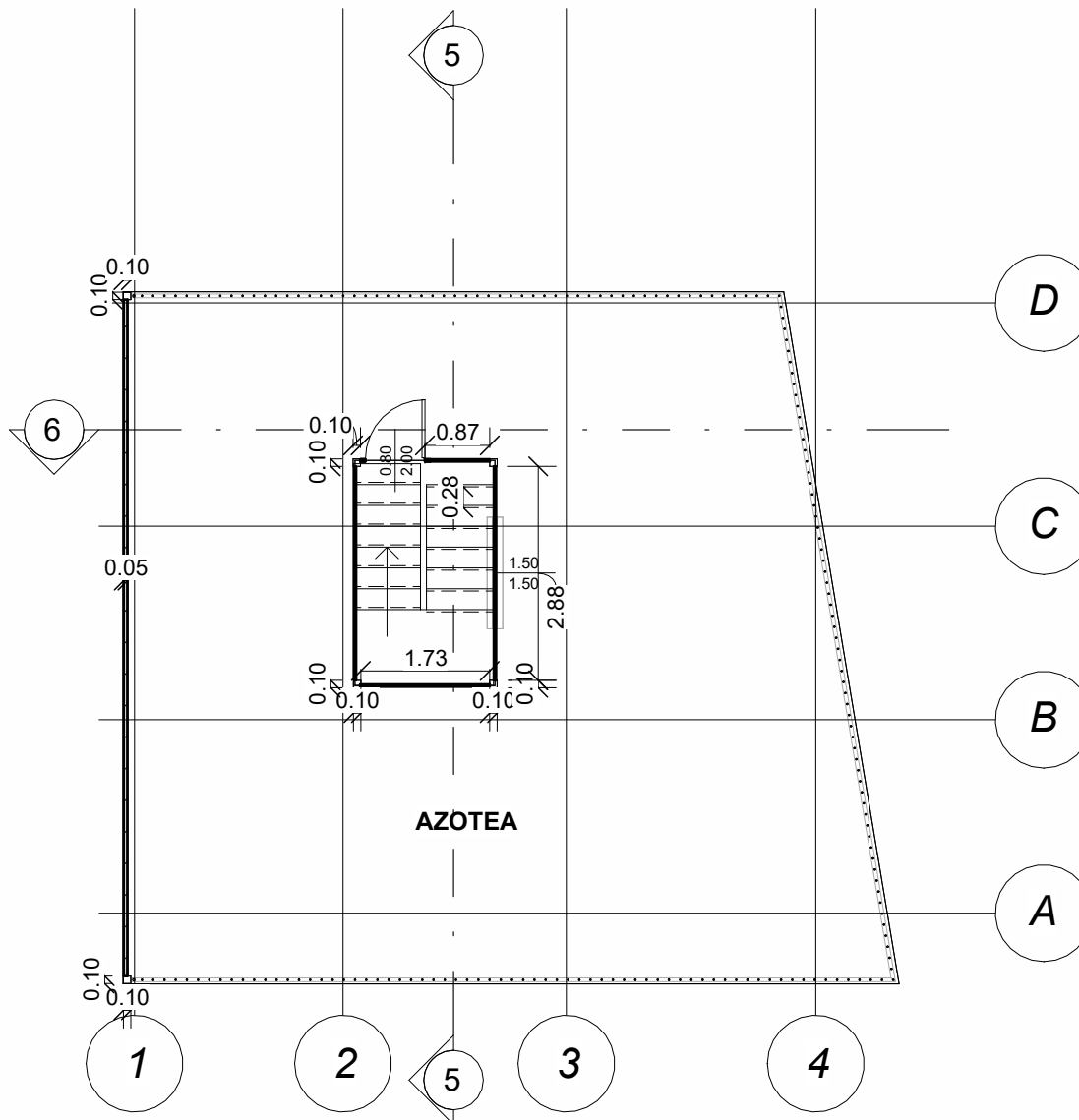
4 Nivel 3 A101 1:100
