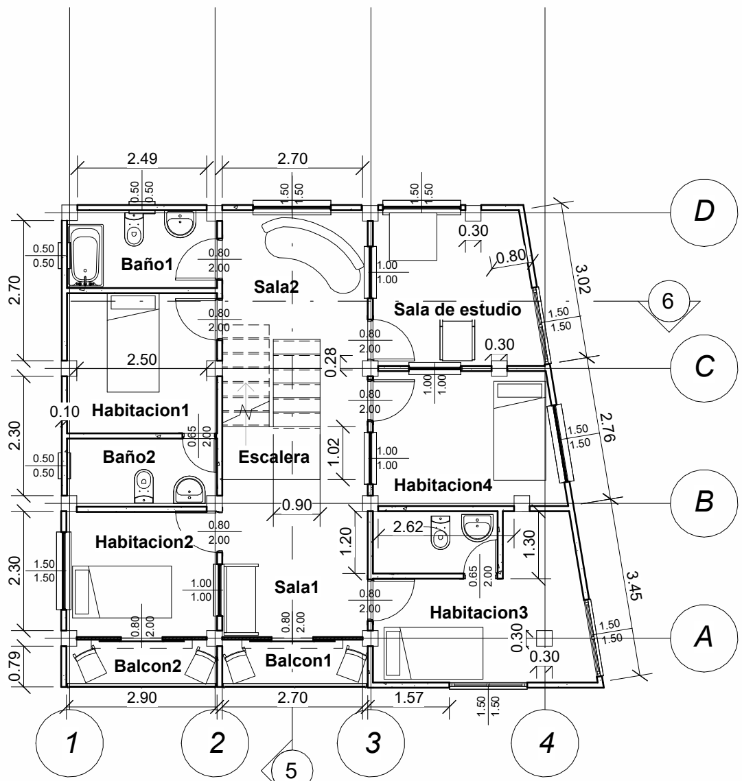
3 Nivel 2 A101 1:100
