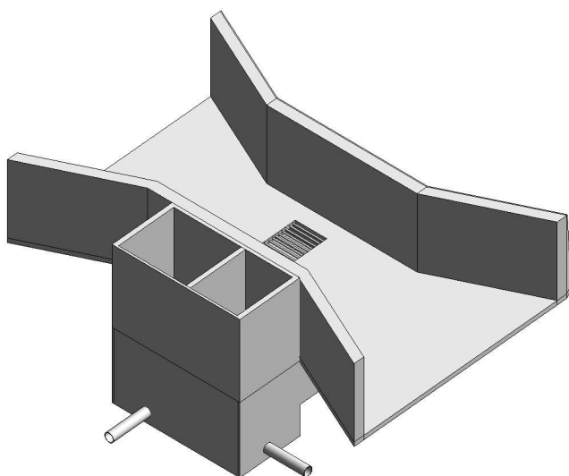
4 Vista isométrica. A102
