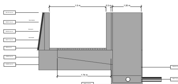
3 Vista en perfil. A102 1:5
