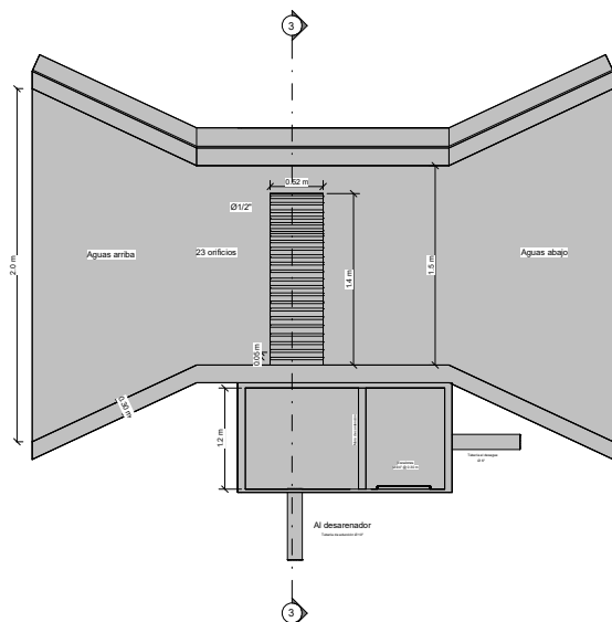
6 Vista en planta. A102 1:5
