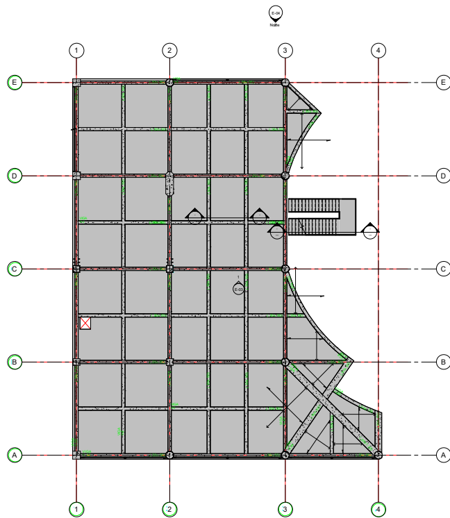
① Encofrado nivel 01 1 : 100
